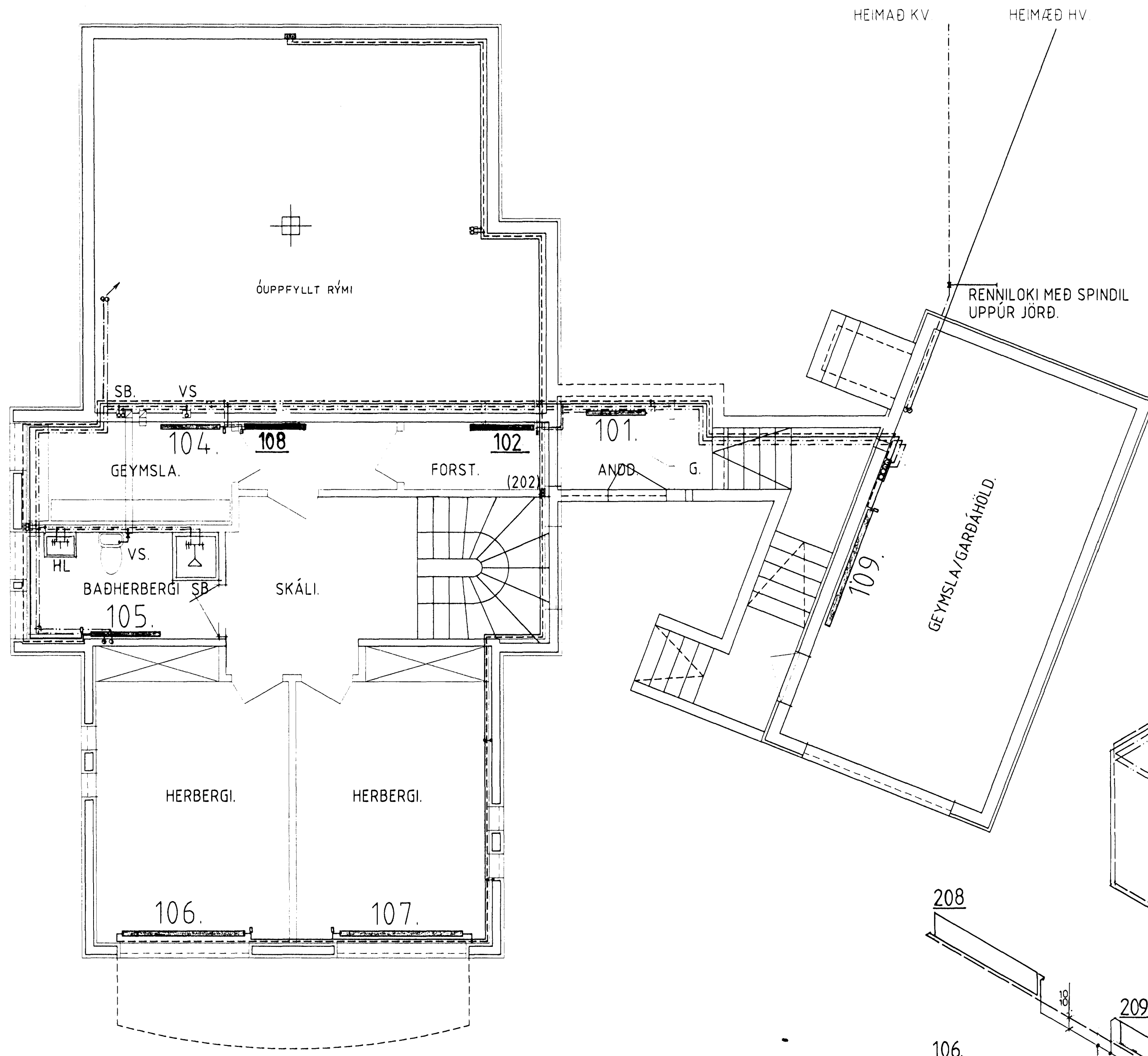
GRUNNMYND 1-HÆÐAR
