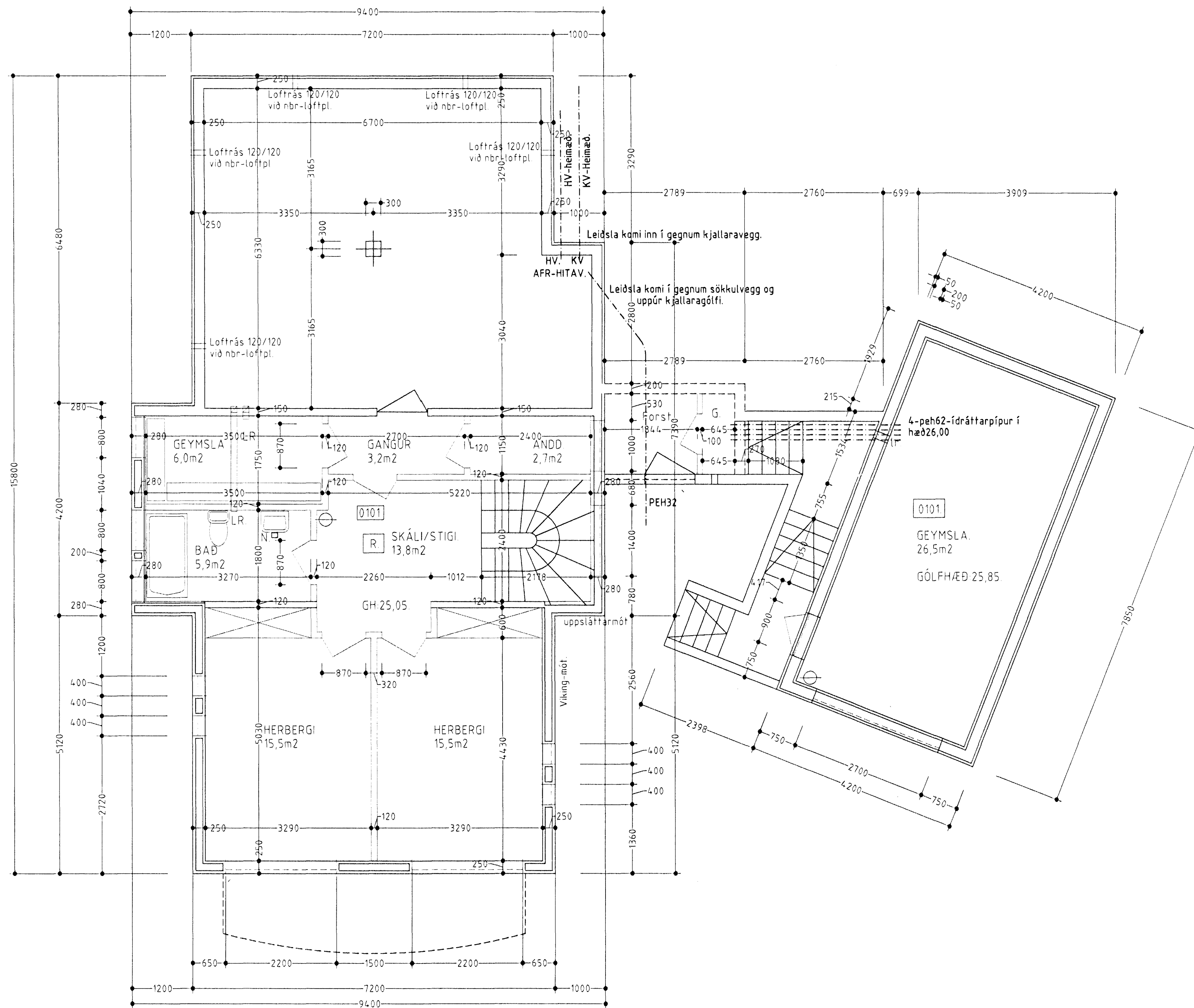
GRUNNMYND 1HÆÐAR.
