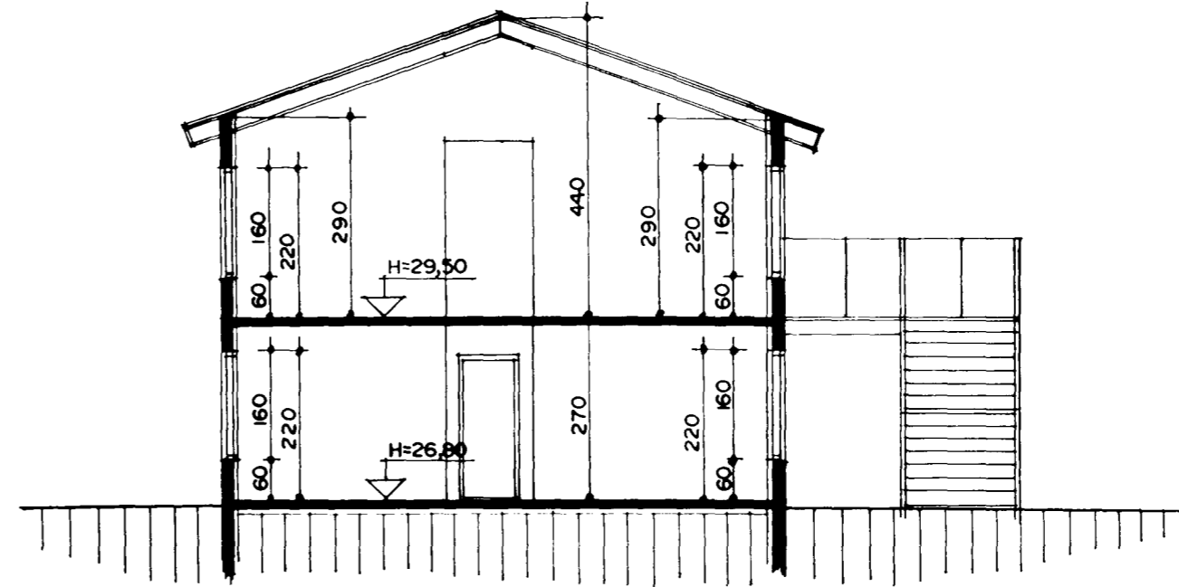
SNEIÐING A-A MKV. 1:100.
