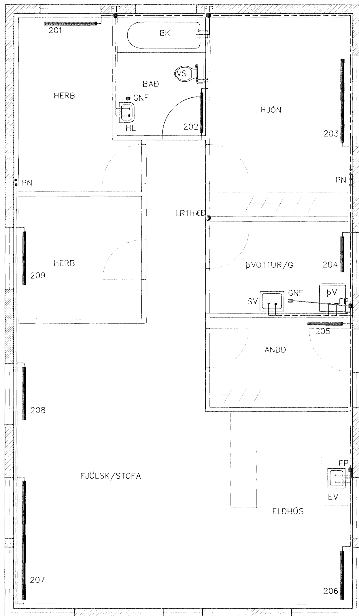
GRUNNMYND 2 HÆÐAR 1:50
