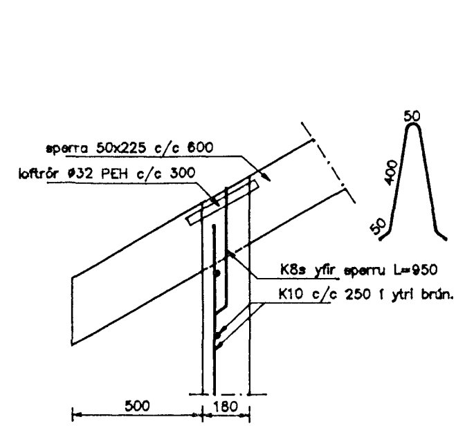
Snið 5-5 Mkv. 1:20
