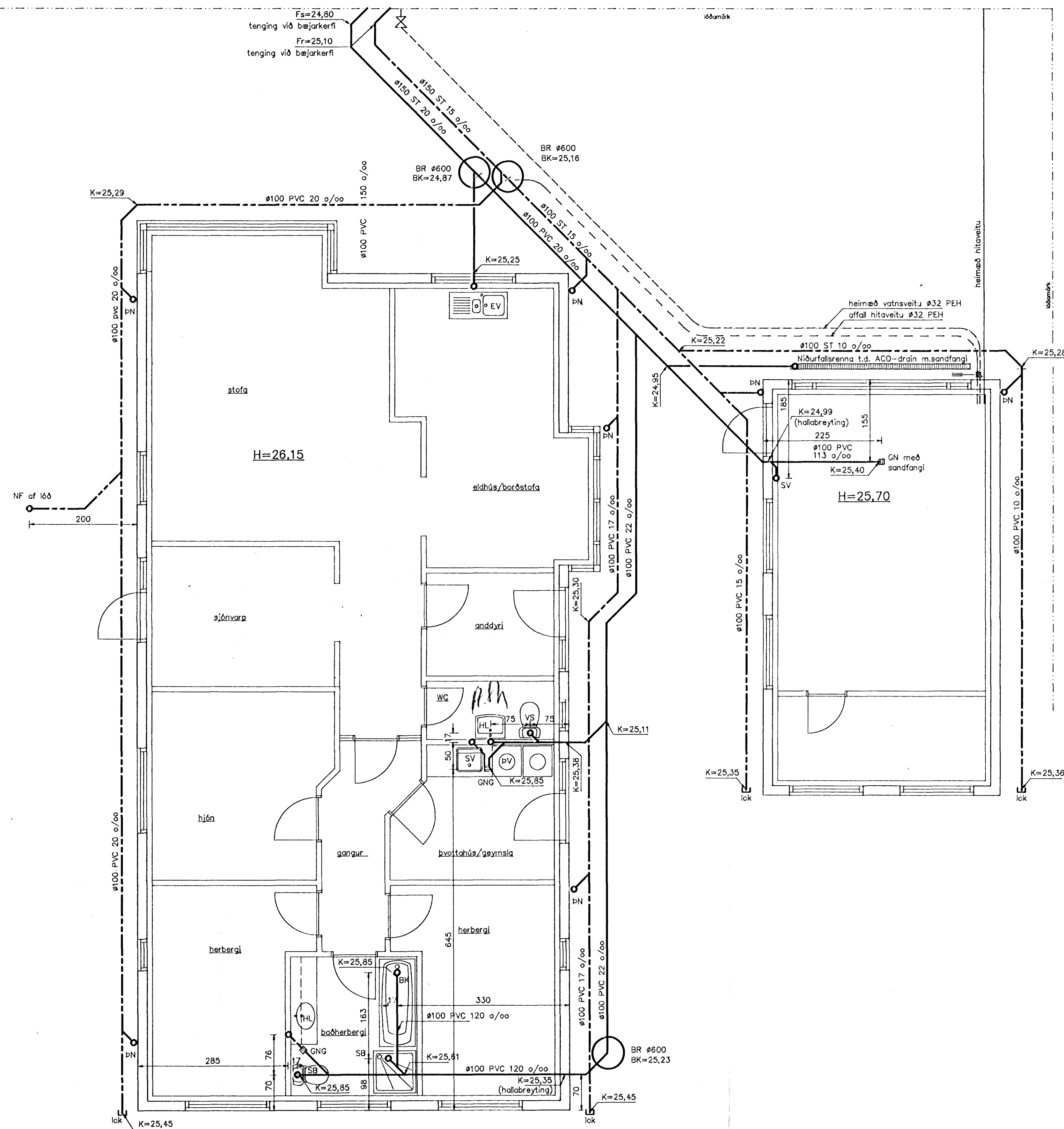
Grunnmynd lagna í jörð mkv. 1:50
