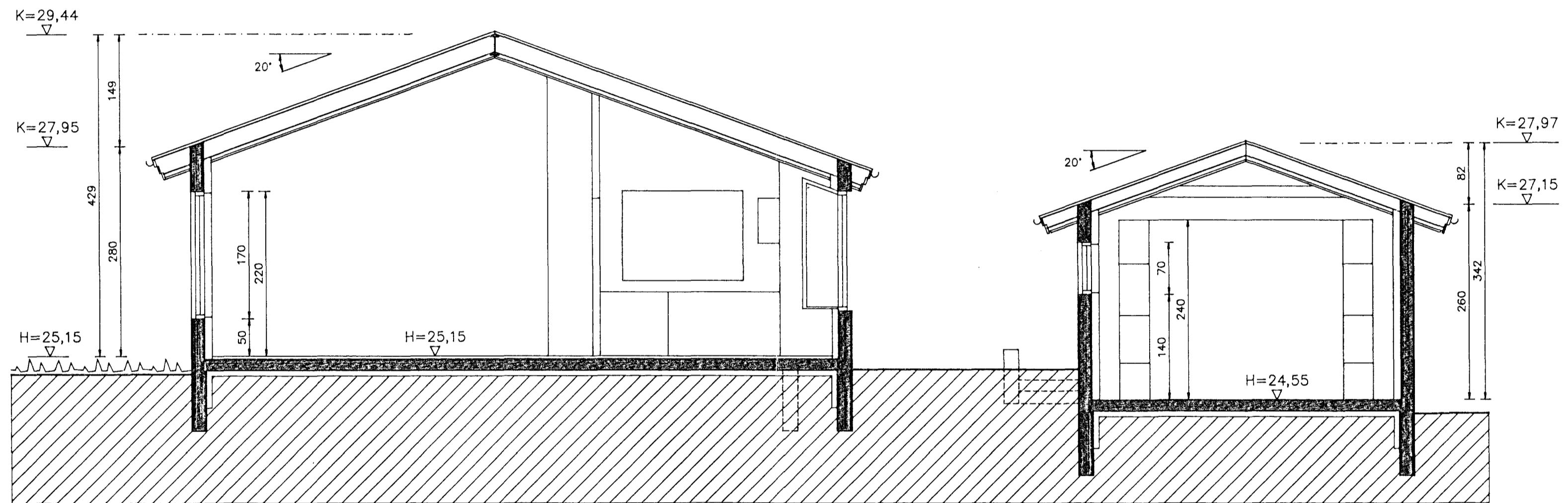
SNID A-A mkv. 1:50
