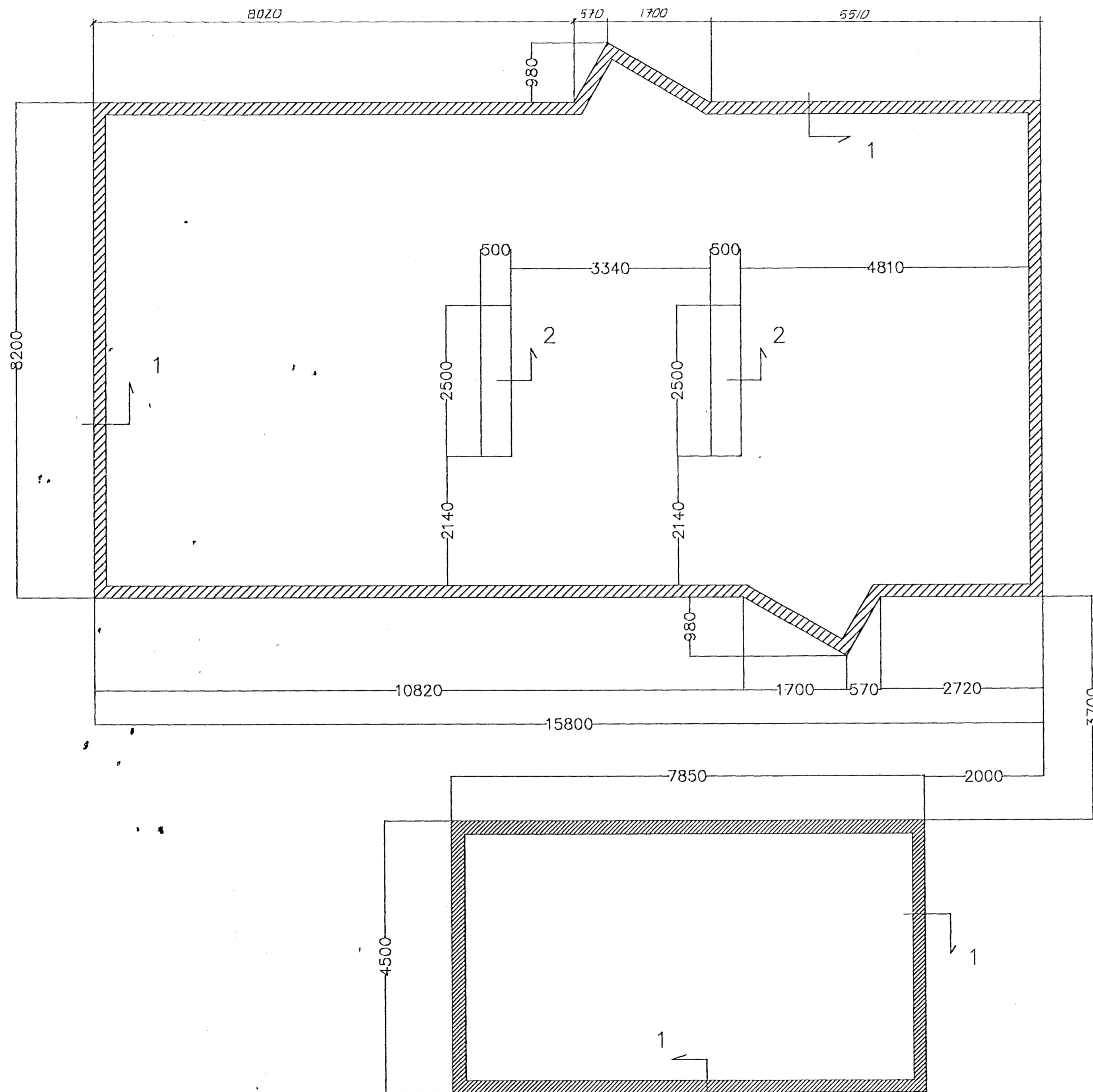
GRUNNMYND 1:50
