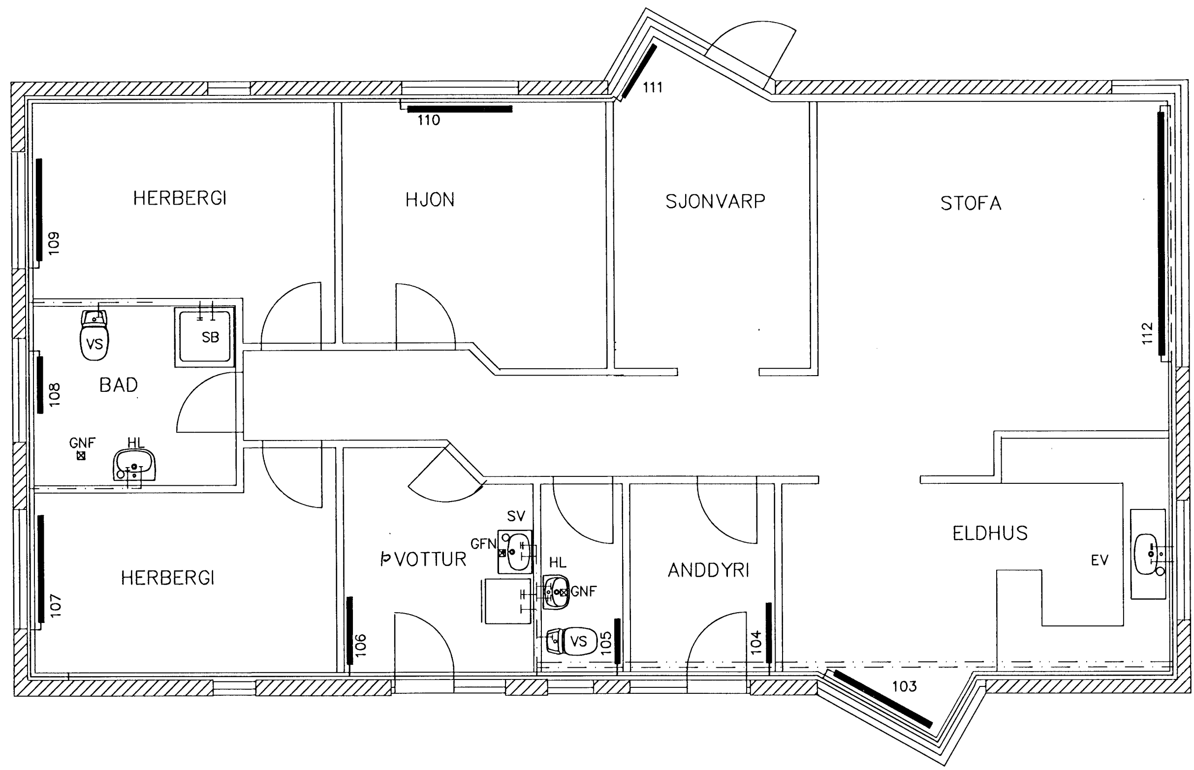
GRUNNMYND 1:50
