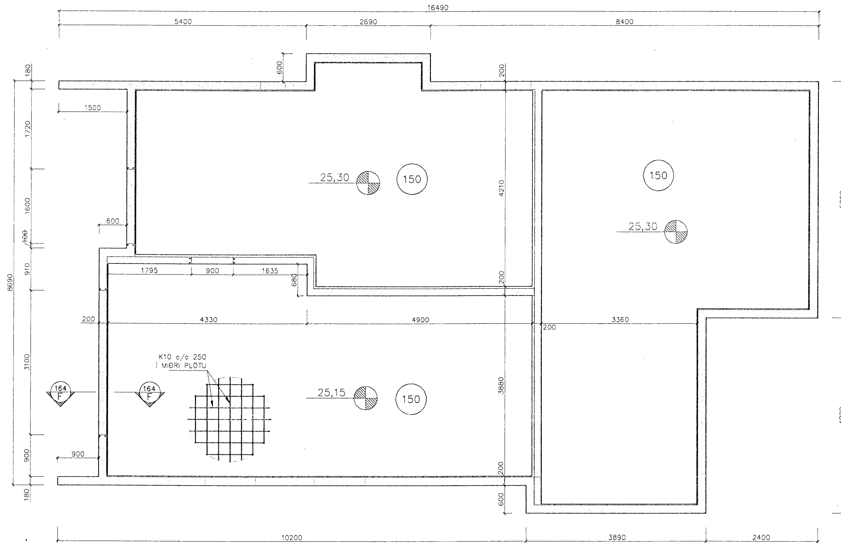
UNDIRSTÖÐUVEGGIR Mkv. 1:50
