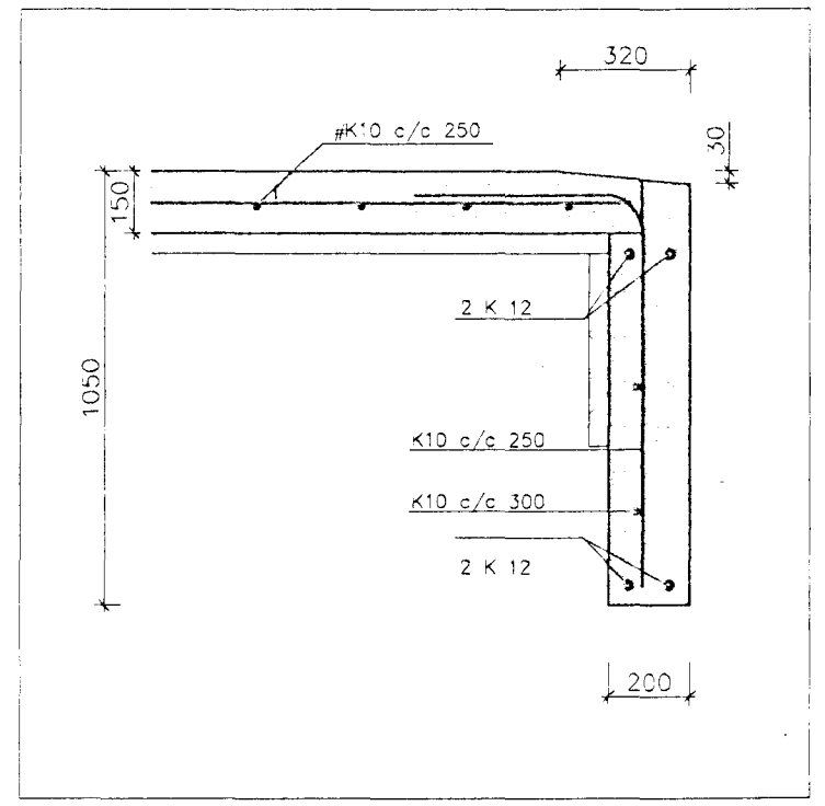
SNID F-F Mkv. 1:20
