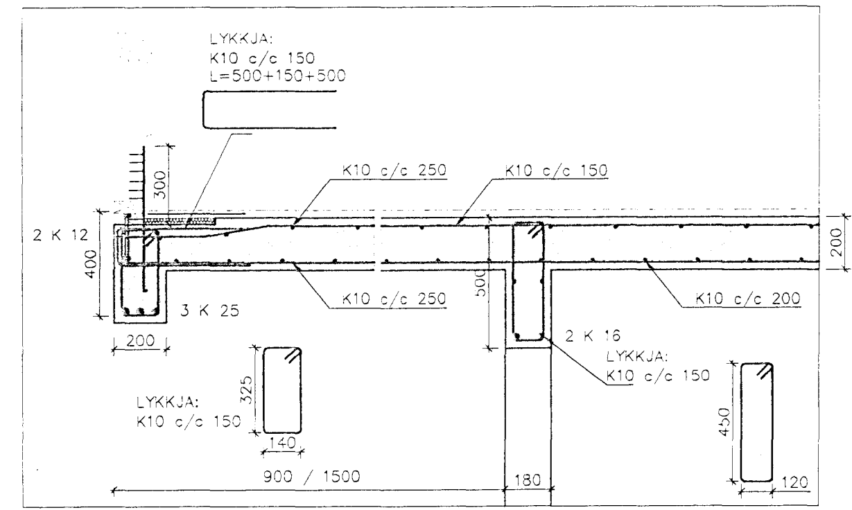
SNID E-E Mkv. 1:20
