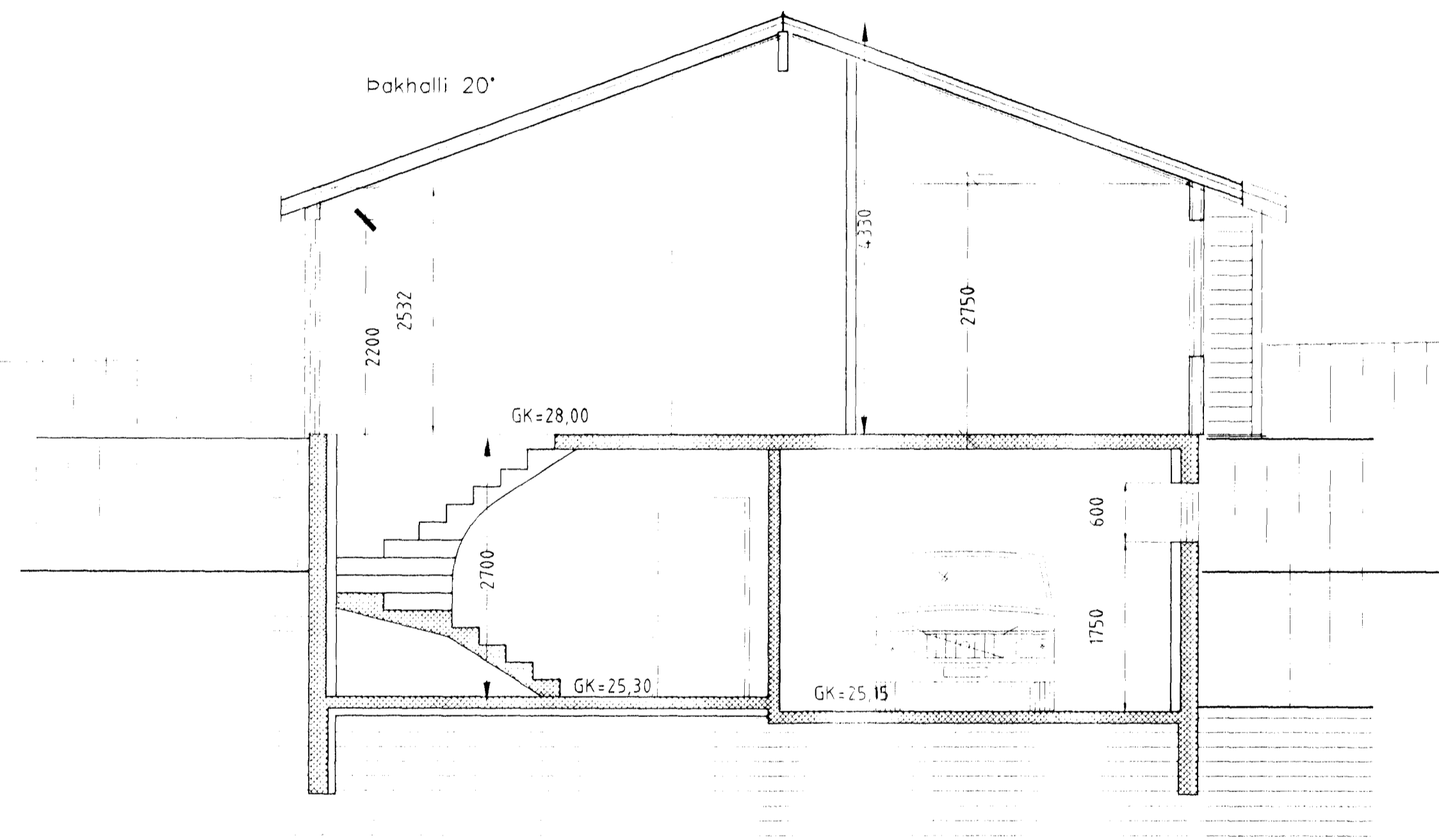
SNIÐ C-C
