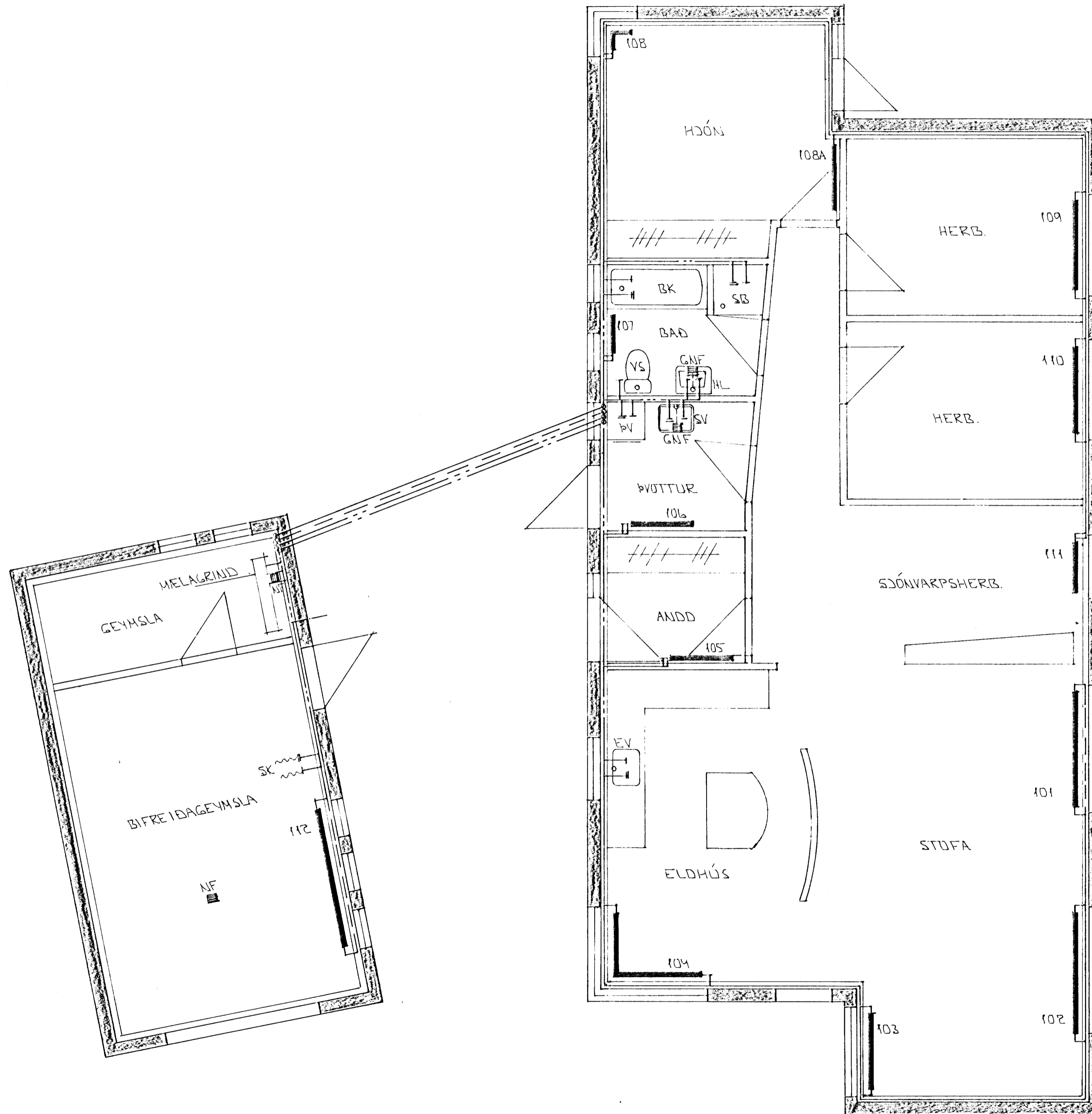
GRUNNMYND 1:50
