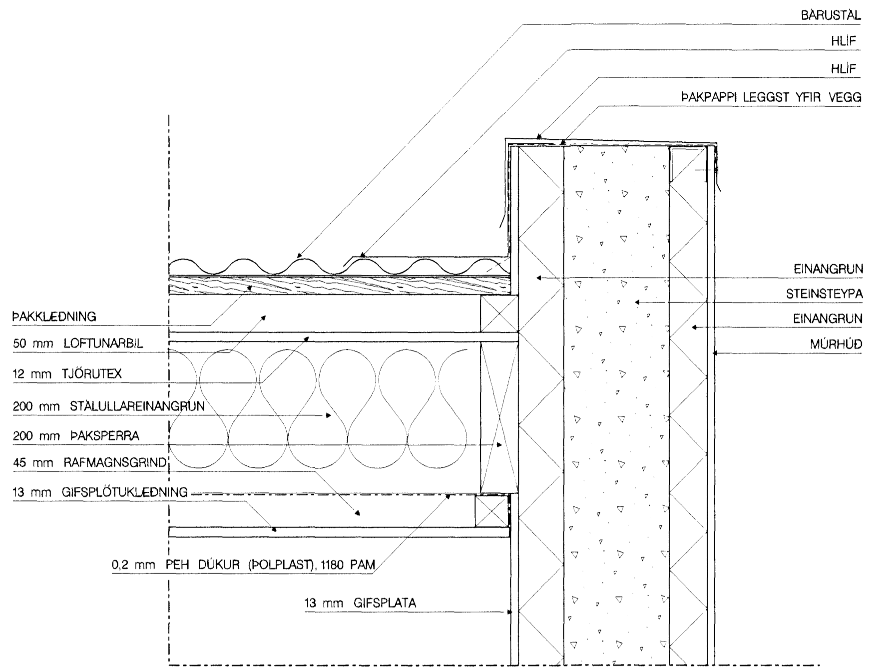
I LÓDRÉTT DEILI - GAFLVEGGUR VIÐ ÞAK MKV. 1:5
