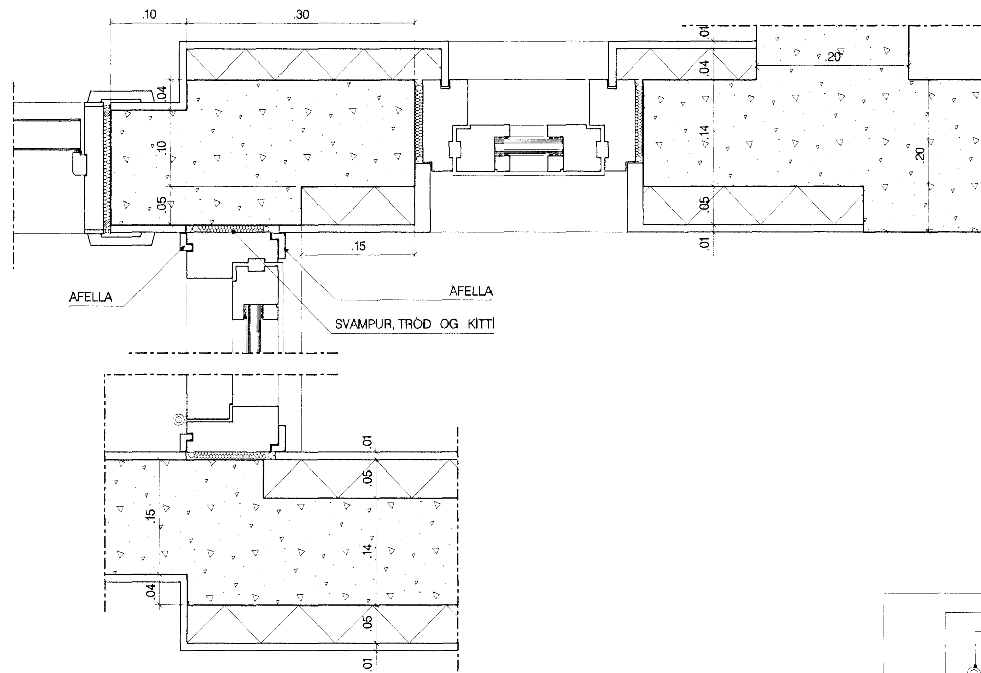
C LARÉTT DEILI 4 MKV. 1:5
