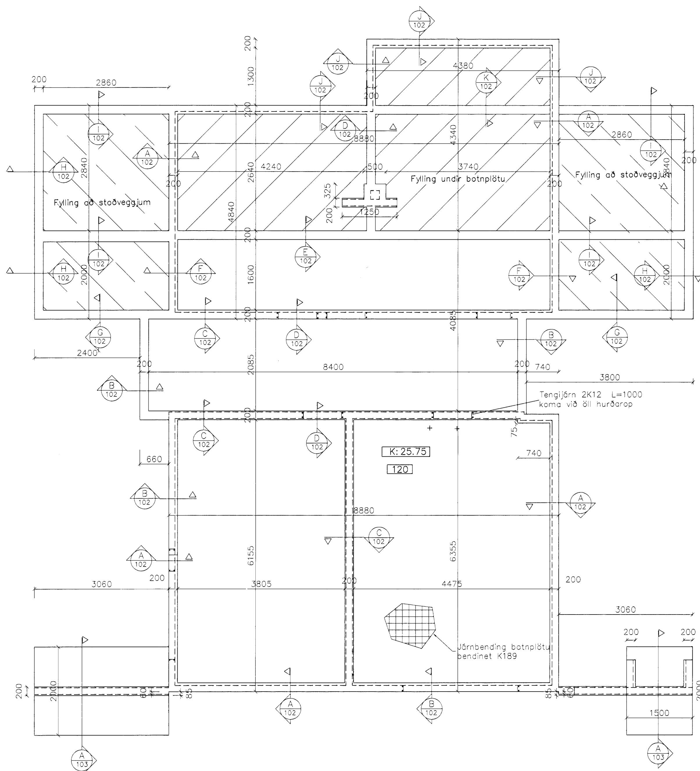
Sökkjar – grunnmynd 1:50
