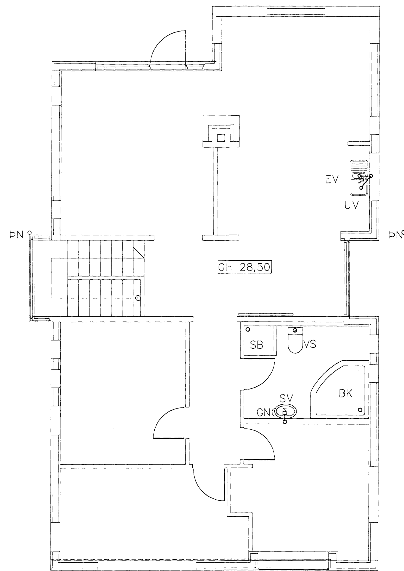
1.hæð grunnmynd 1:50
