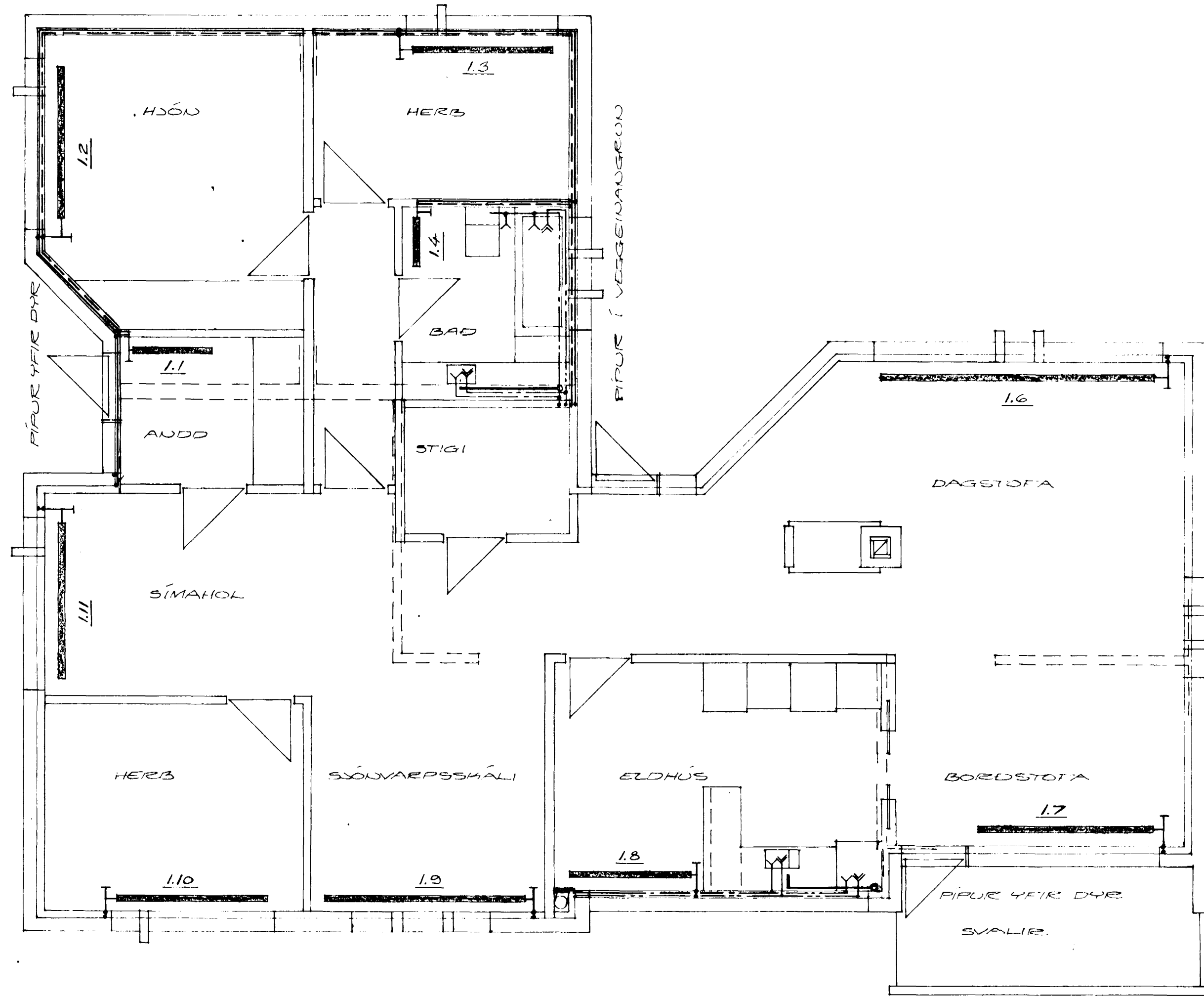
GRUNNMYND HÉÐAR M=1:50
