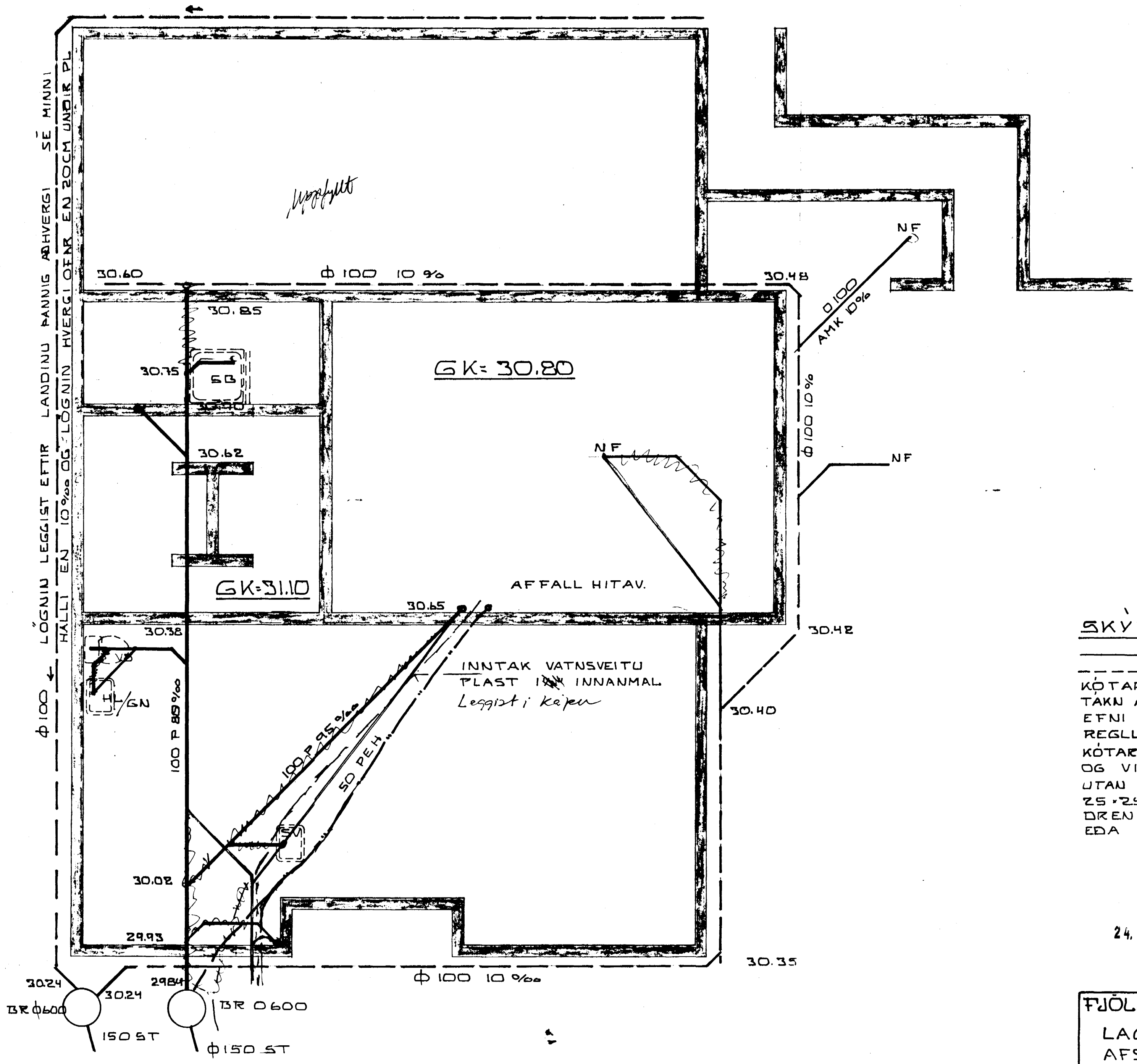
GRUNNMYND UNDIRSTÖÐUR 1:50
