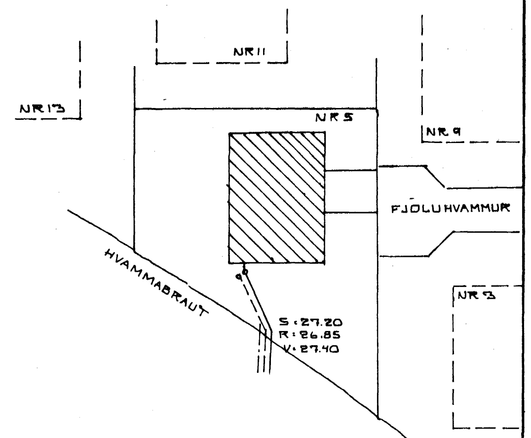
AFSTÖÐUMYND 1:500
