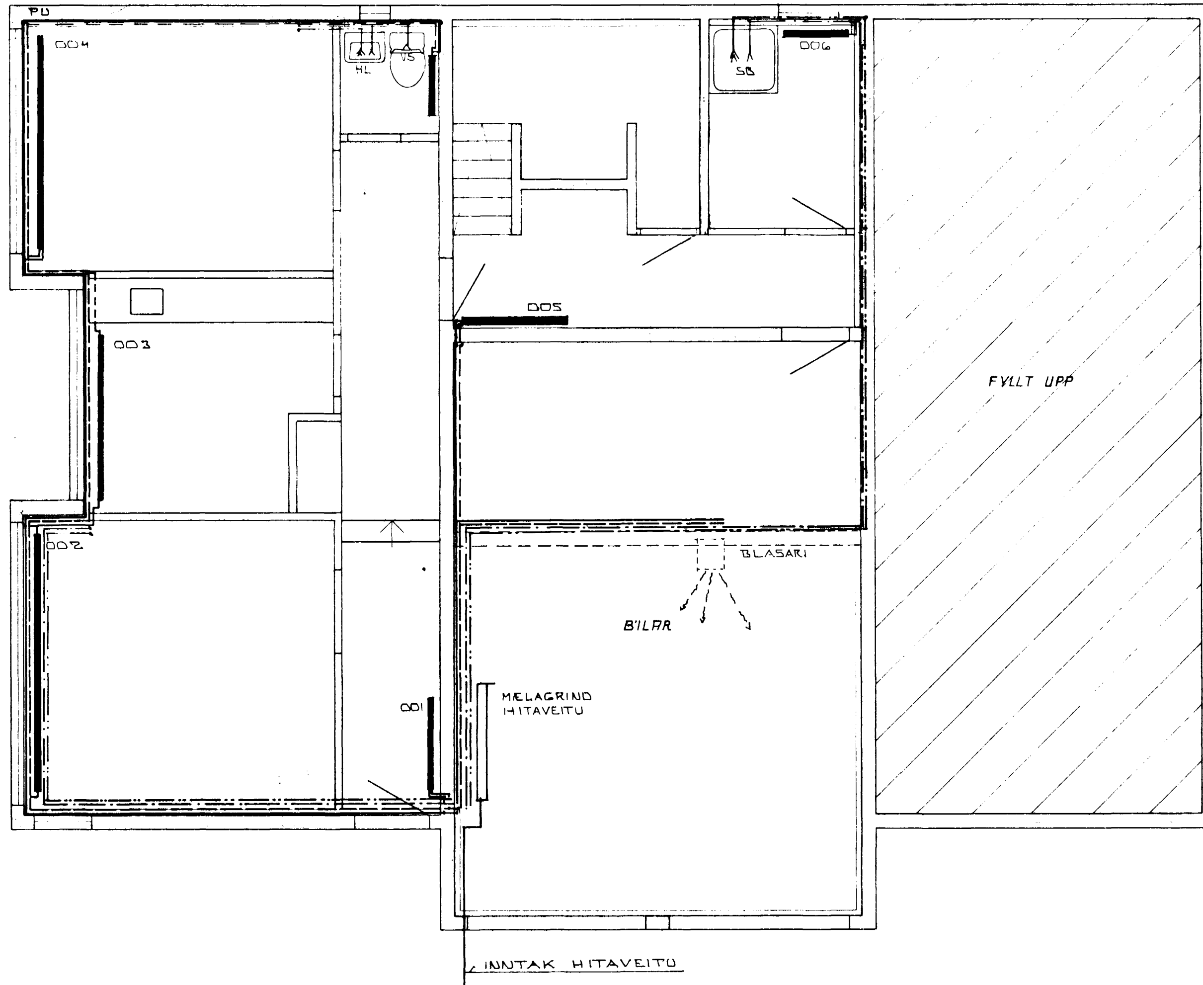
GRUNNMYND KJALLARA 1:50
