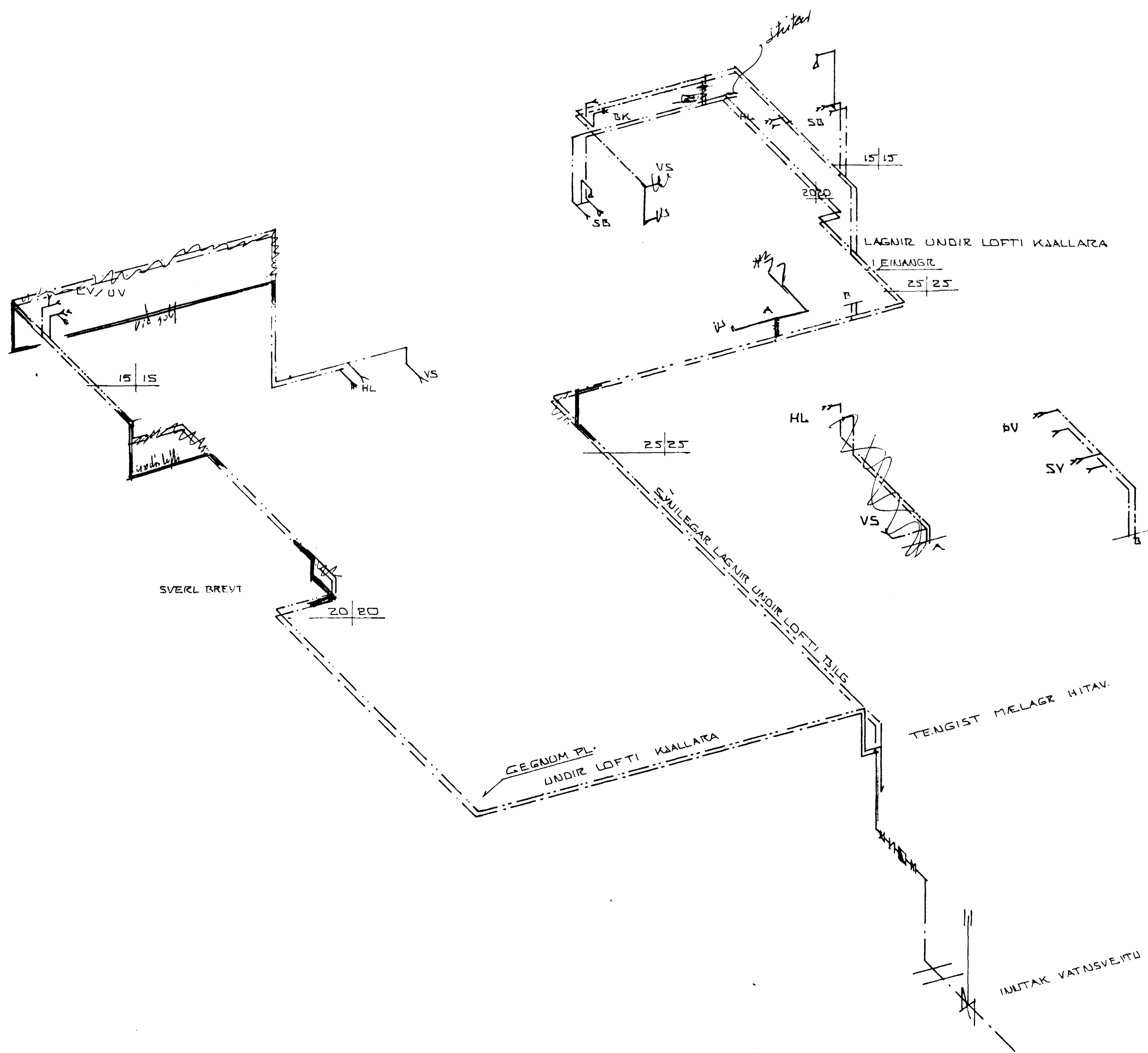
RÜMMYND VATNSLAGNA ~1:50
