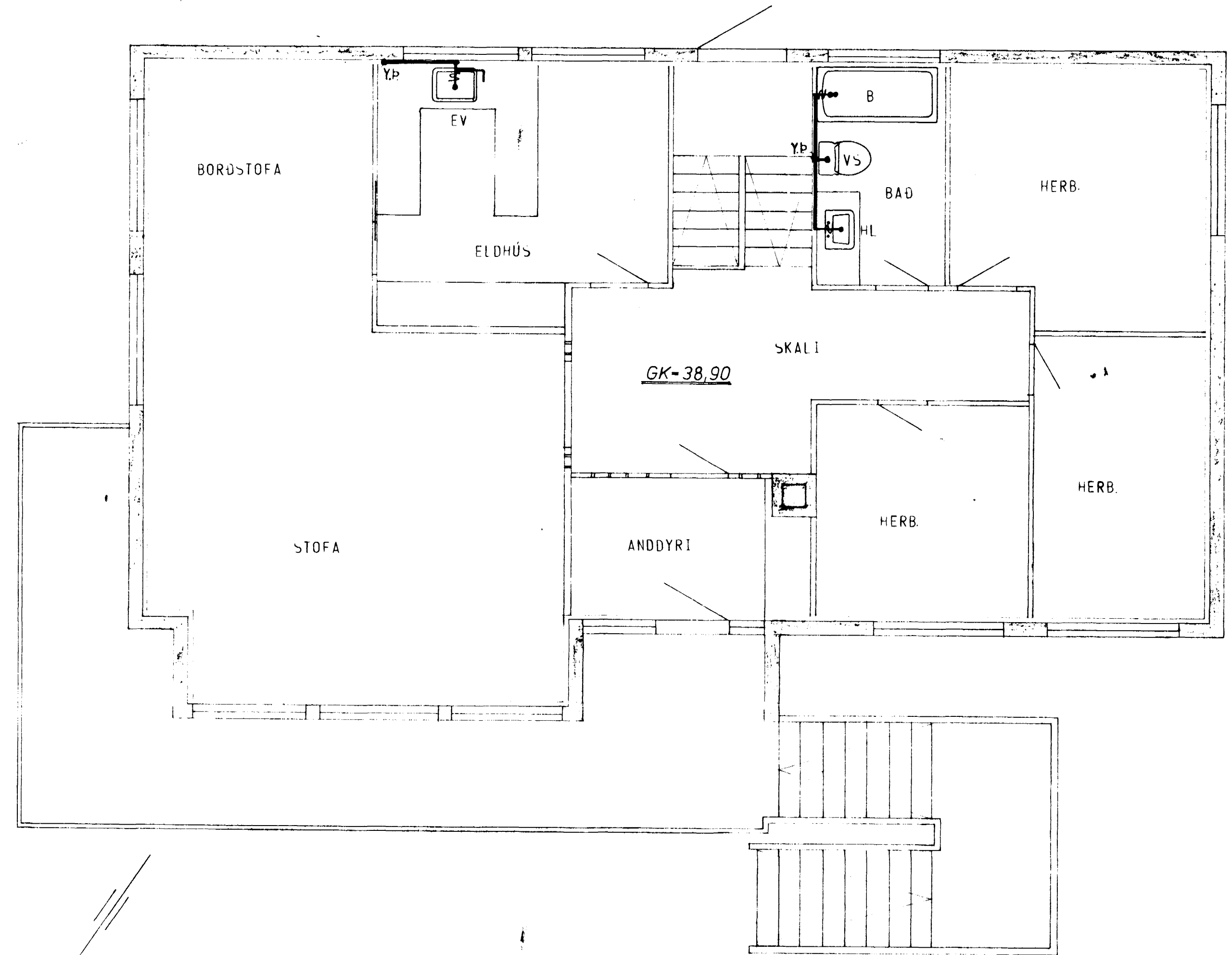
GRUNNMYND HÆÐAR 1:50
