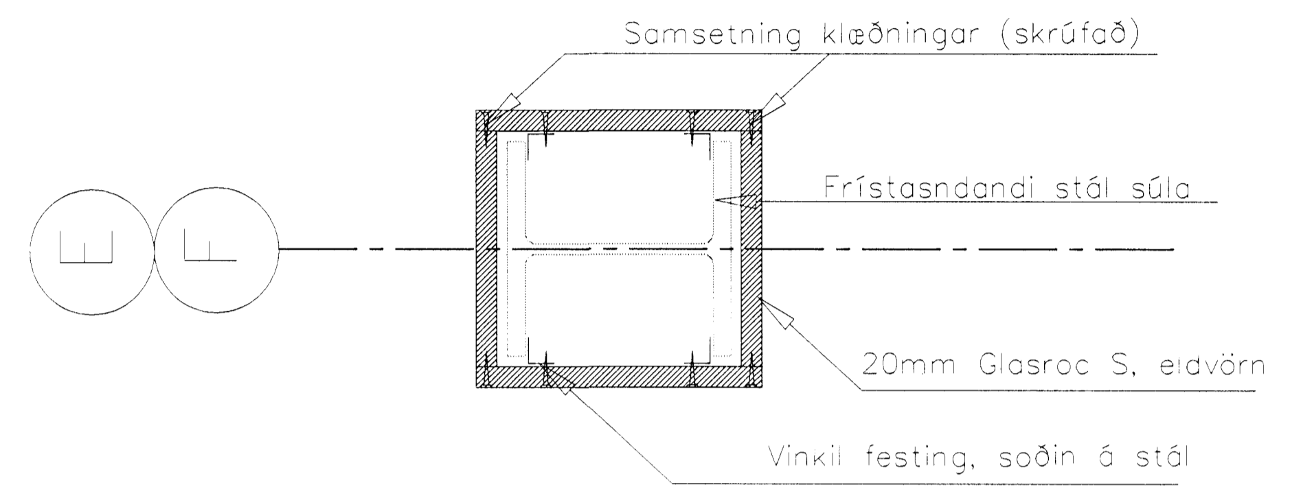
Súlu-deili /1:5
