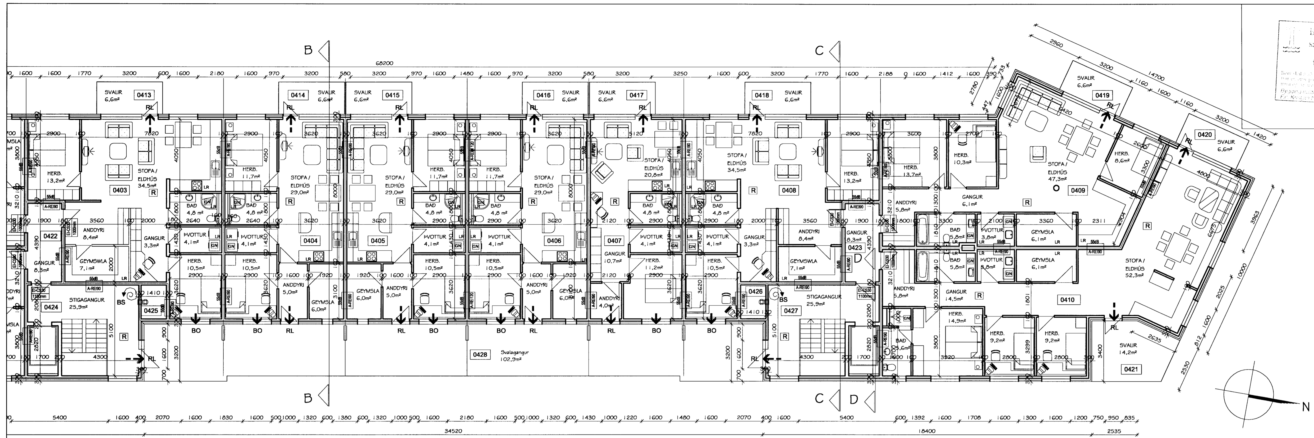
GRUNNMYND 4. HÆÐ NORÐUR
