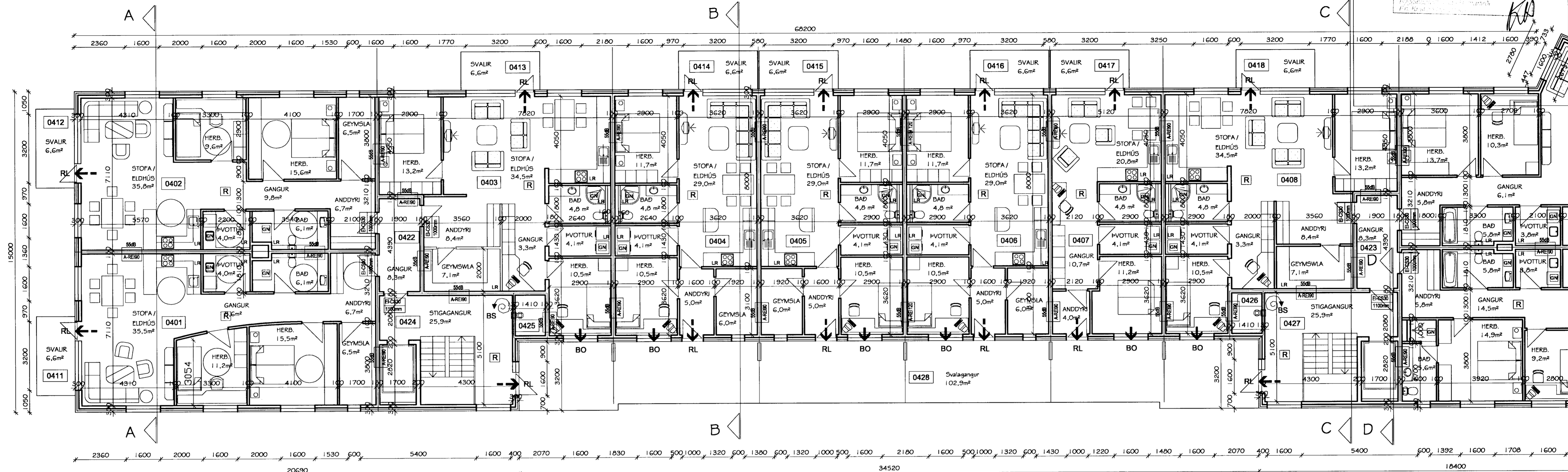
4. HÆÐ 1080,5 m 2 GRUNNMYND 4. HÆÐ
