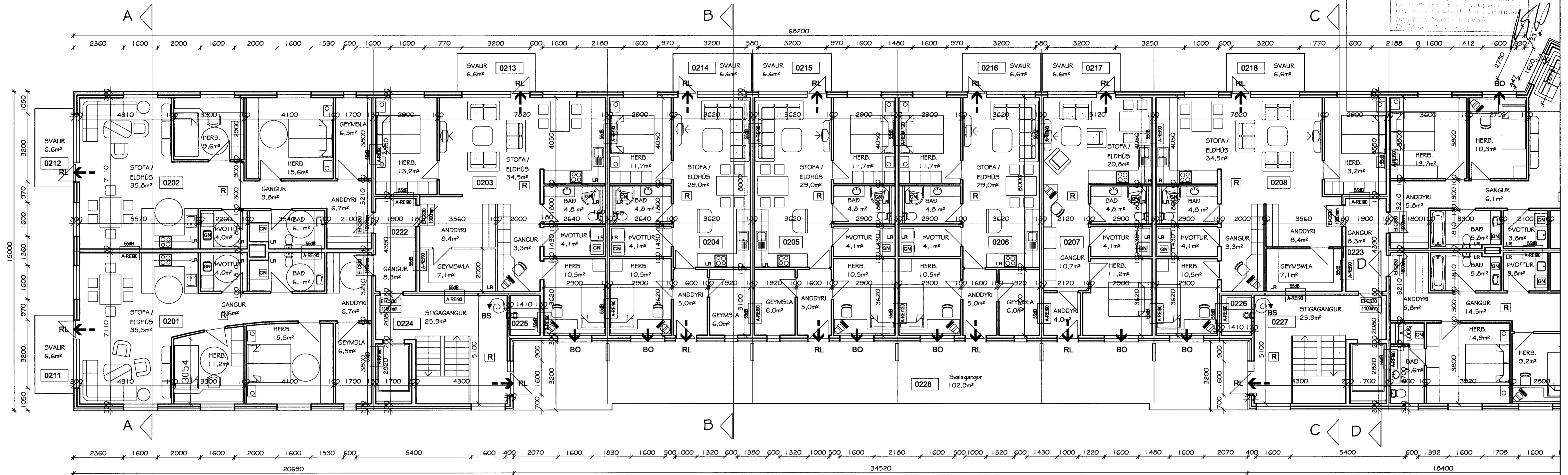
2. HÆÐ 1080,5 m 2 GRUNNMYND 2. HÆÐ
