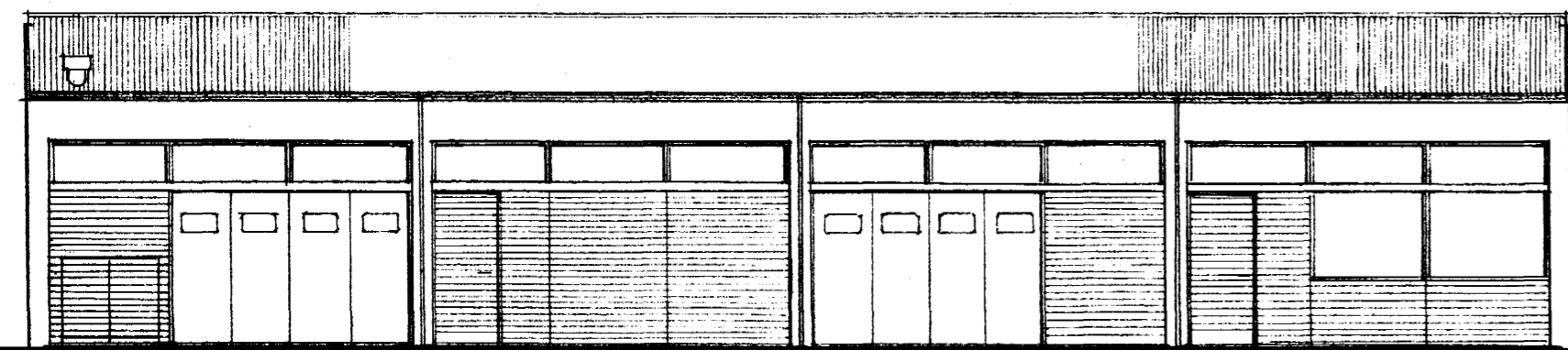
AUSTURHLID M 1:100
