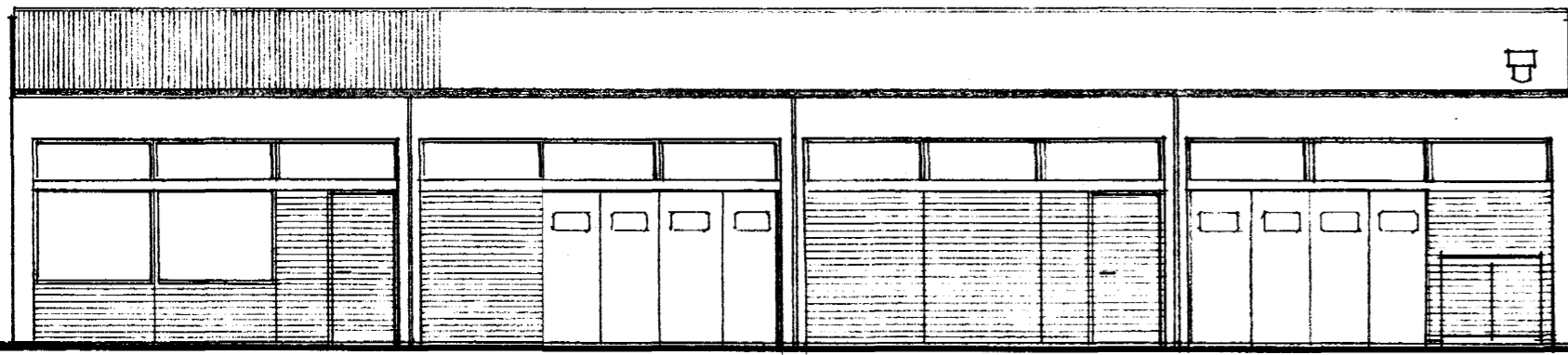
VESTURHLID M 1:100
