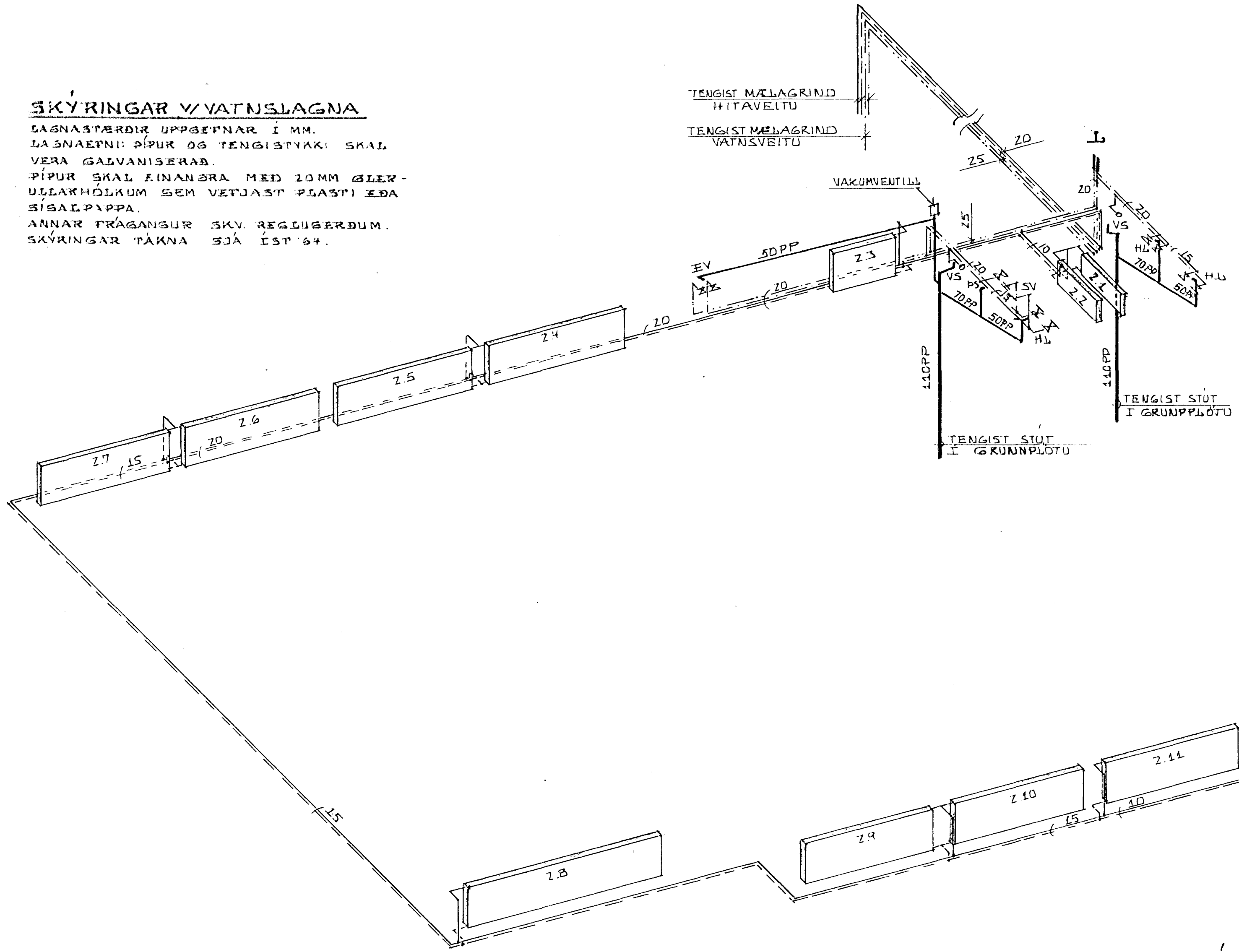
KERFISMYND HITA- OG HREINLÆTISLAGNA 1:50
