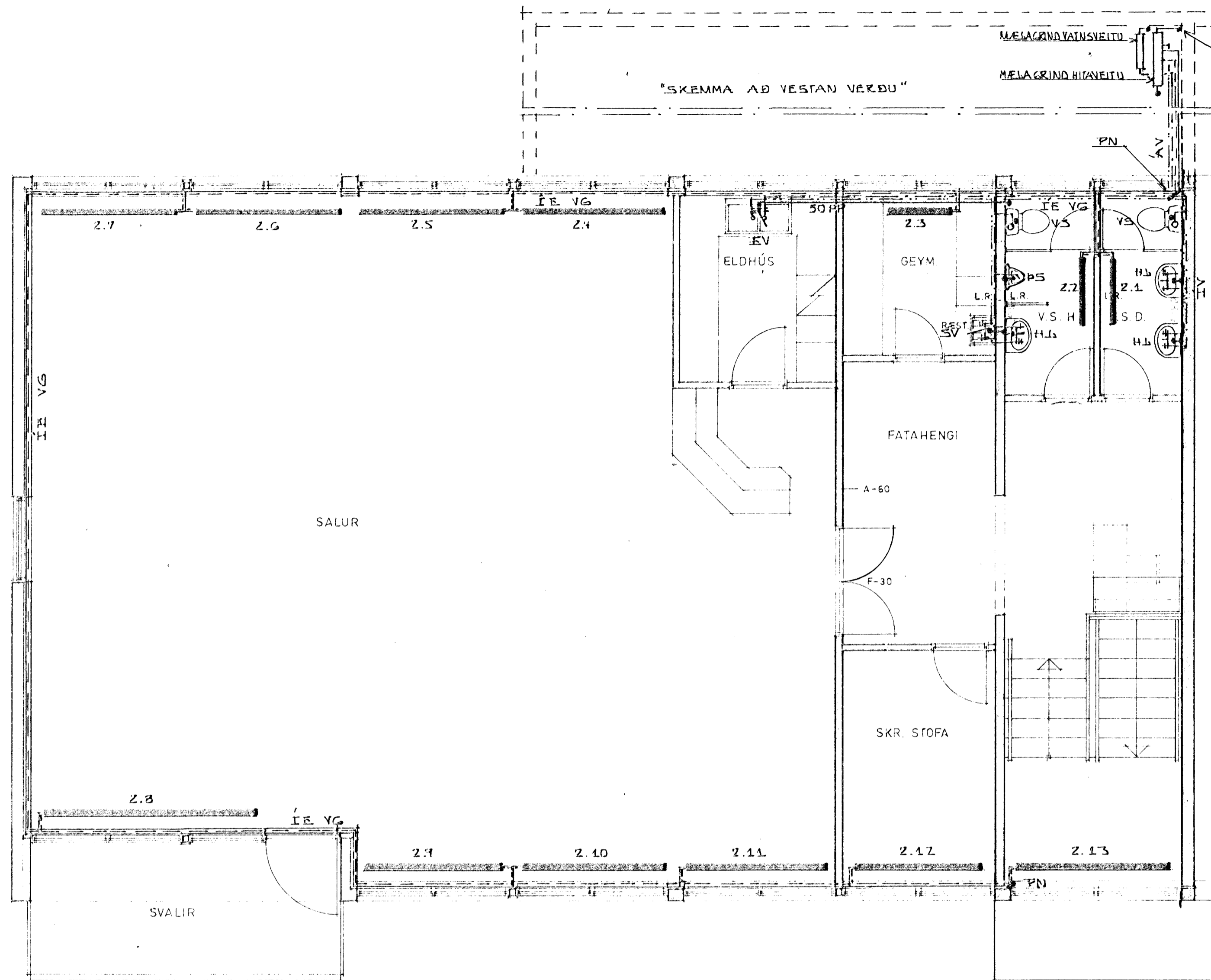
GRUNNMYND EÐRI HÆÐAR 1:50
