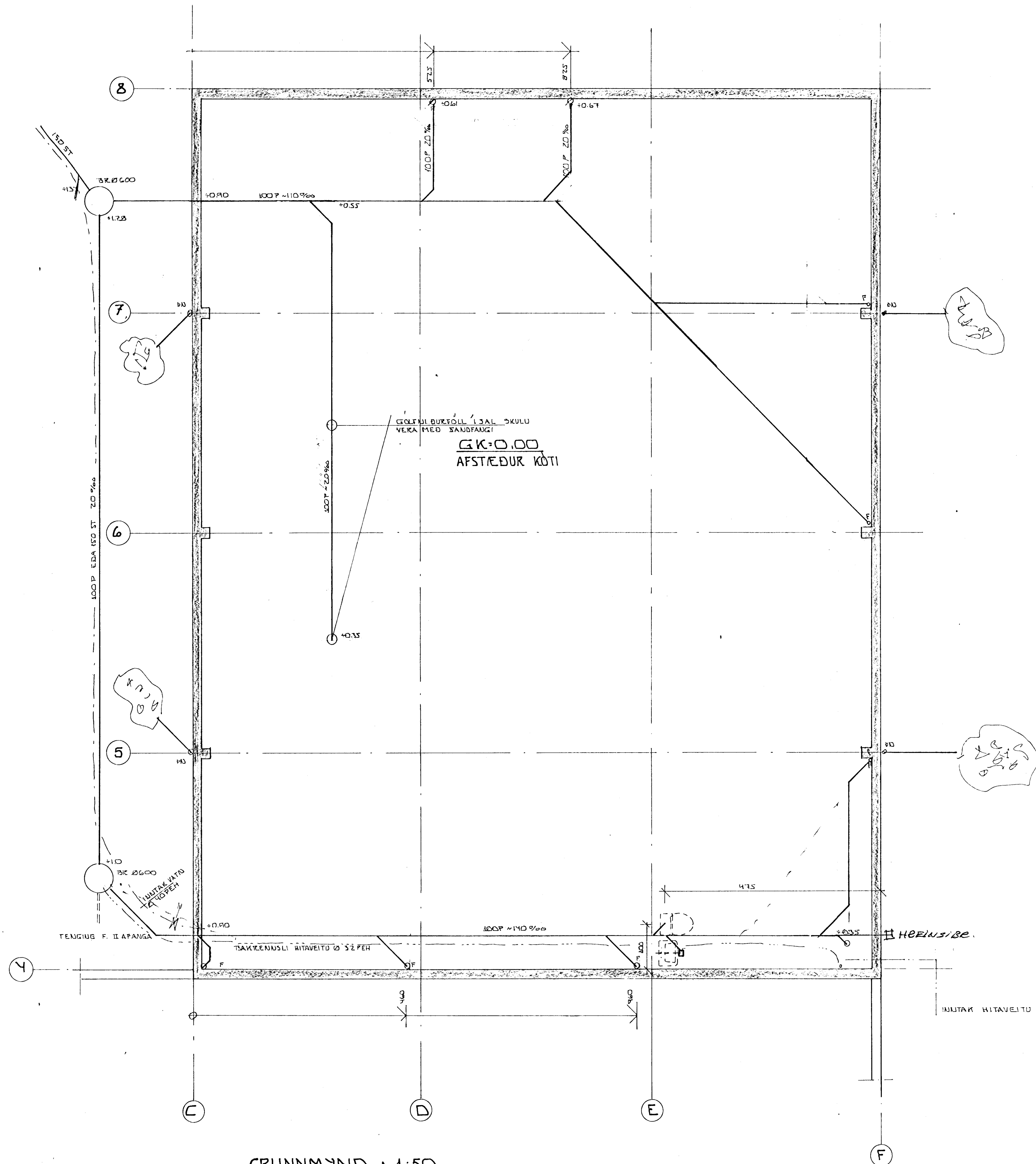
GRUNNMYND - 1:50
