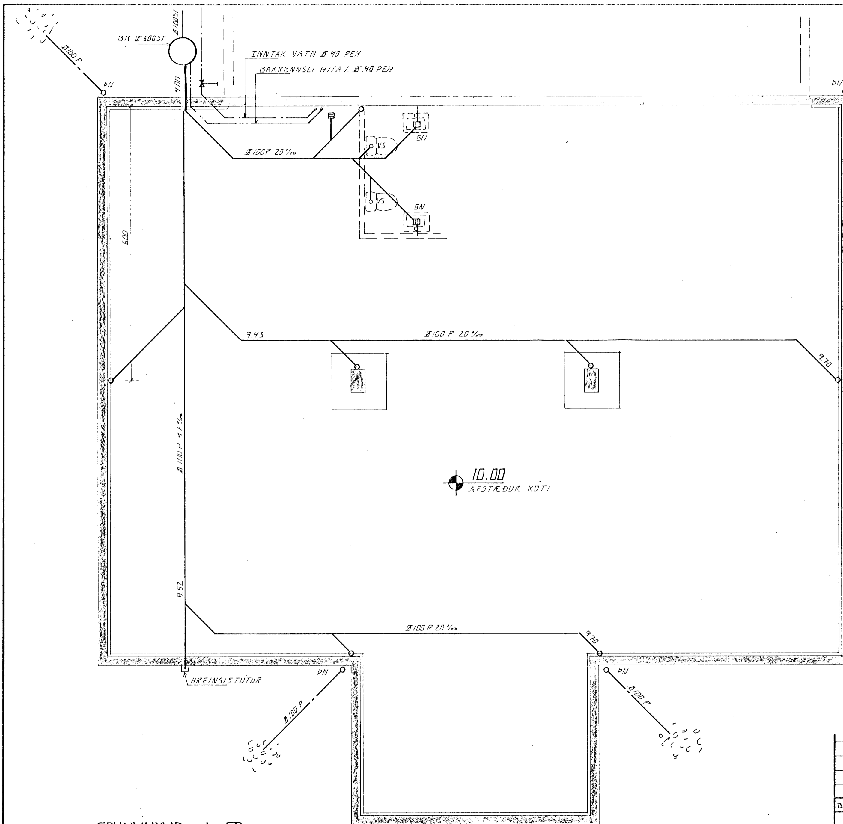
GRUNNMYND - 1:50
