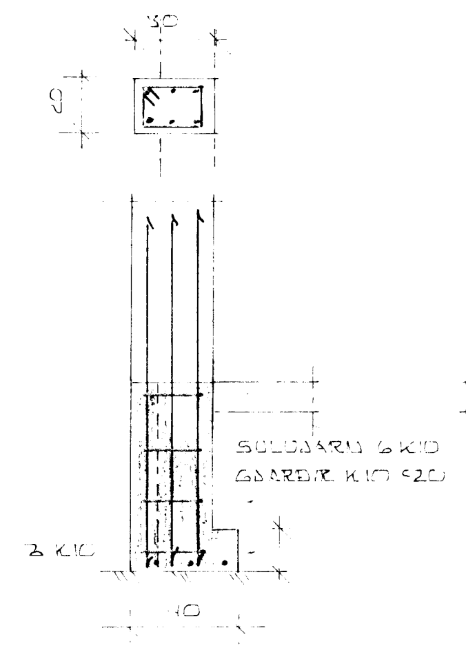
SUIÐ C 1:20
