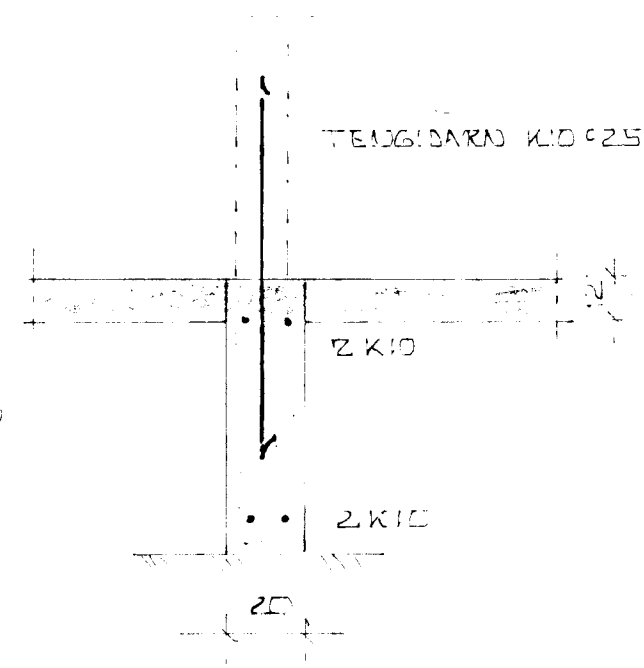
SUIÐ D 1:20
