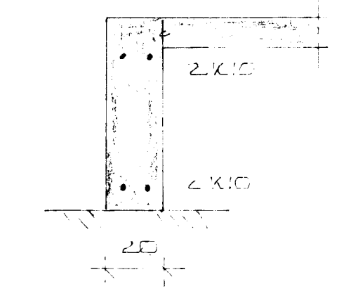
SUIÐ E 1:20
