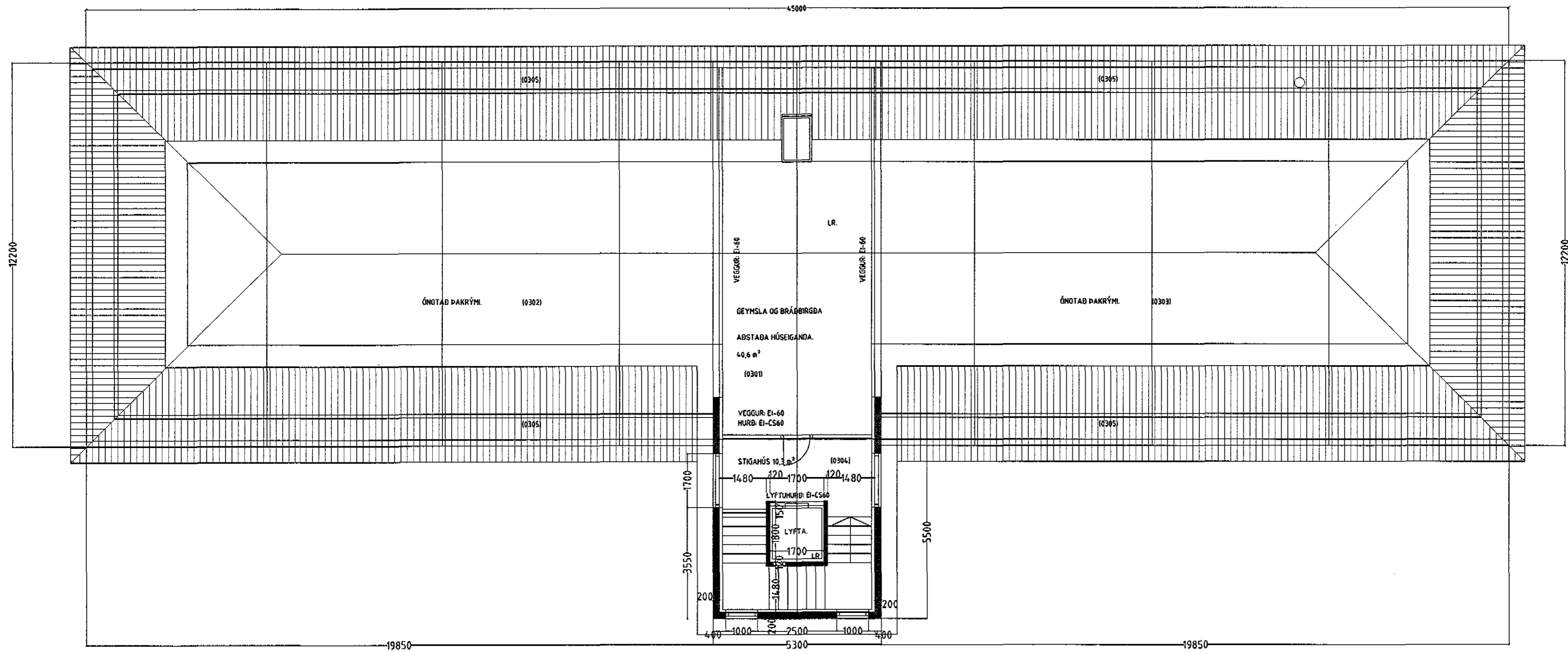
GRUNNMYND ÞAKHÆÐAR. MKV. 1:100.
