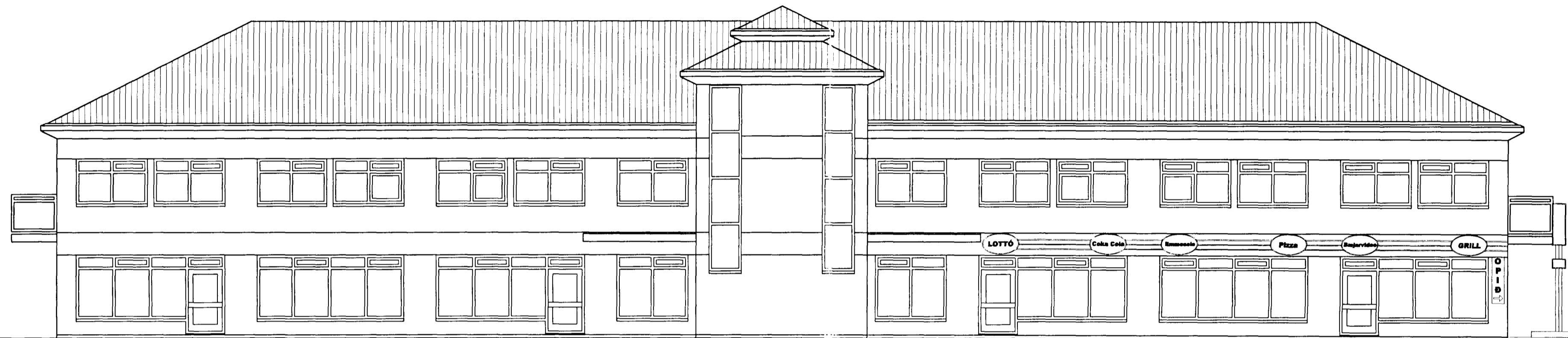
ÚTLIT SUÐUR MKV. 1:100.
