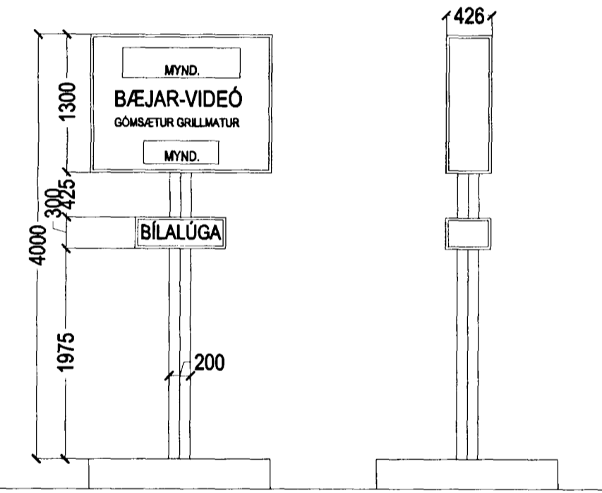
AUGLÝSINGASKILTÍ MKV. 1:50.
