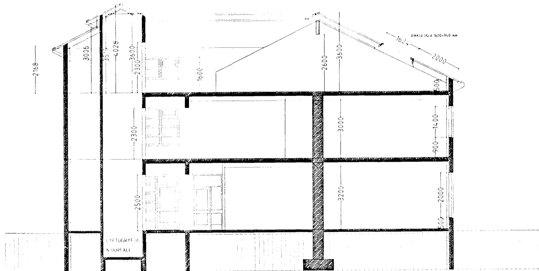
SNIDMYND MKV 1:100
