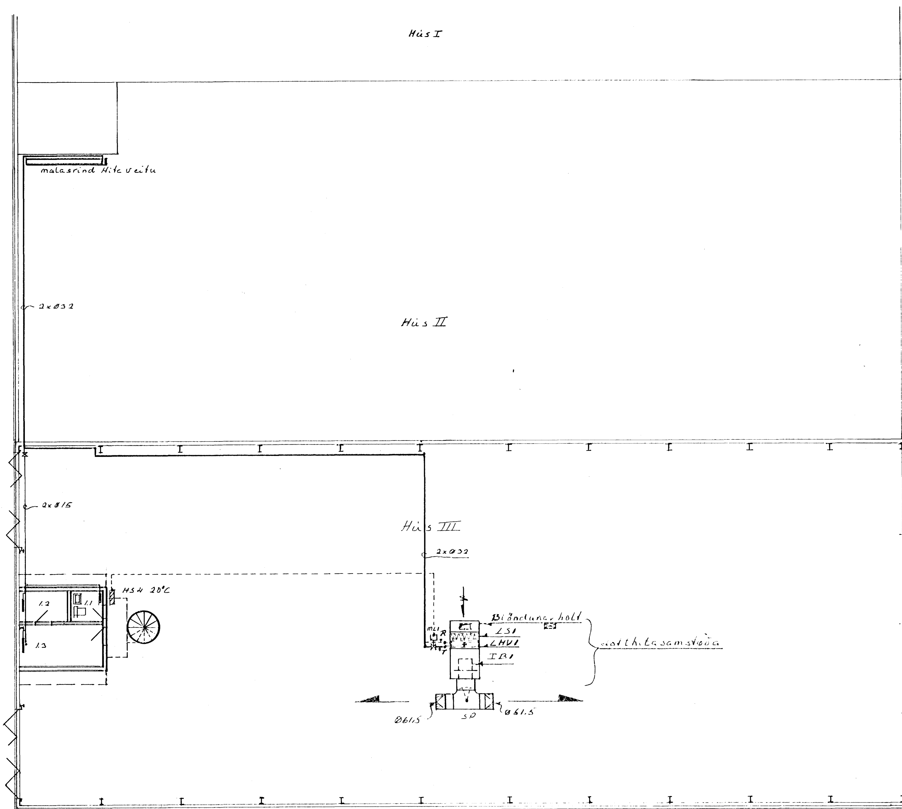
Grunnmynd Hús III 1:100
