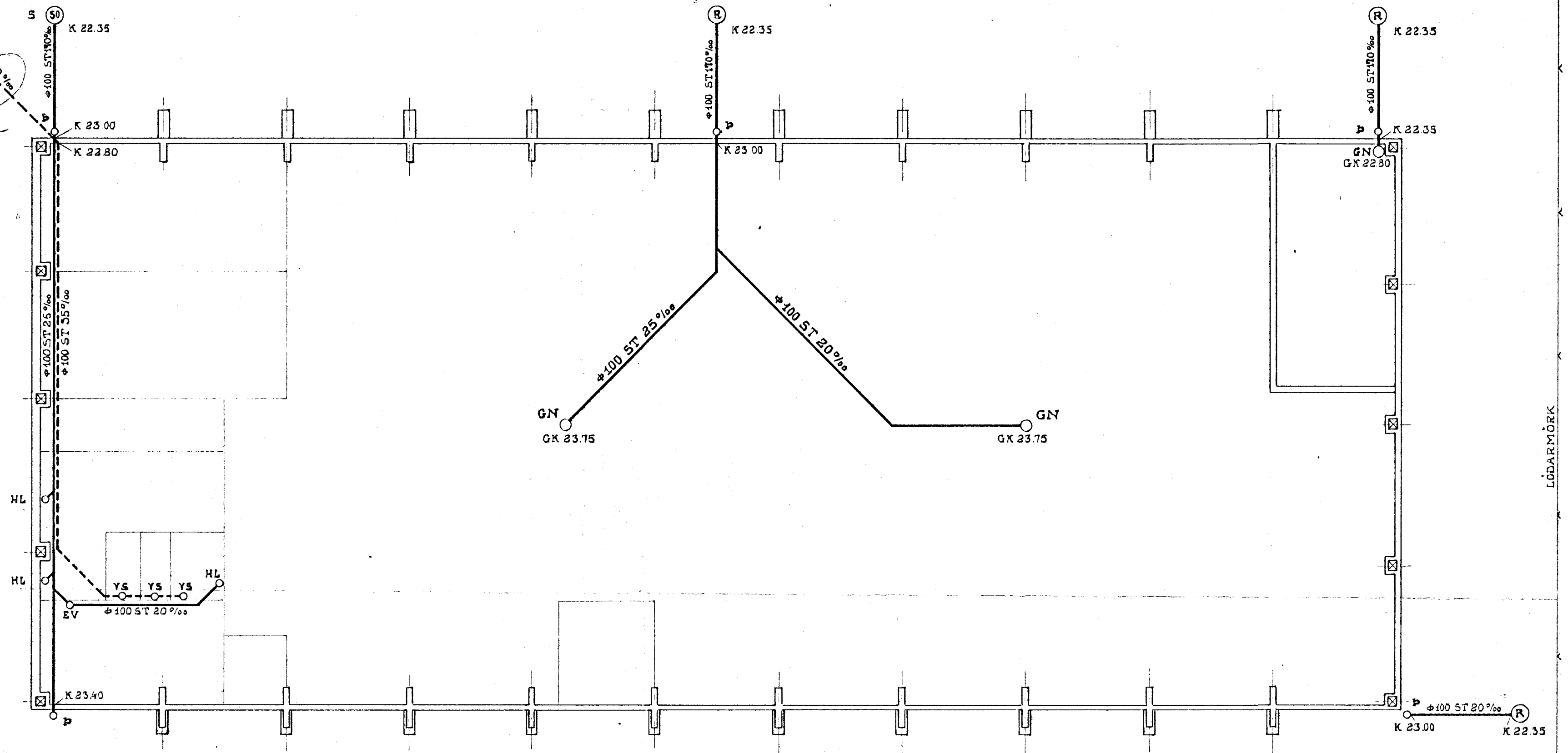
REGNVATNSSVELGUR M=1:20
