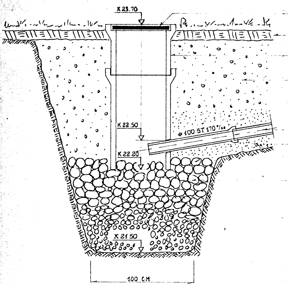
SKOLVATNSSVELGUR M=1:20
