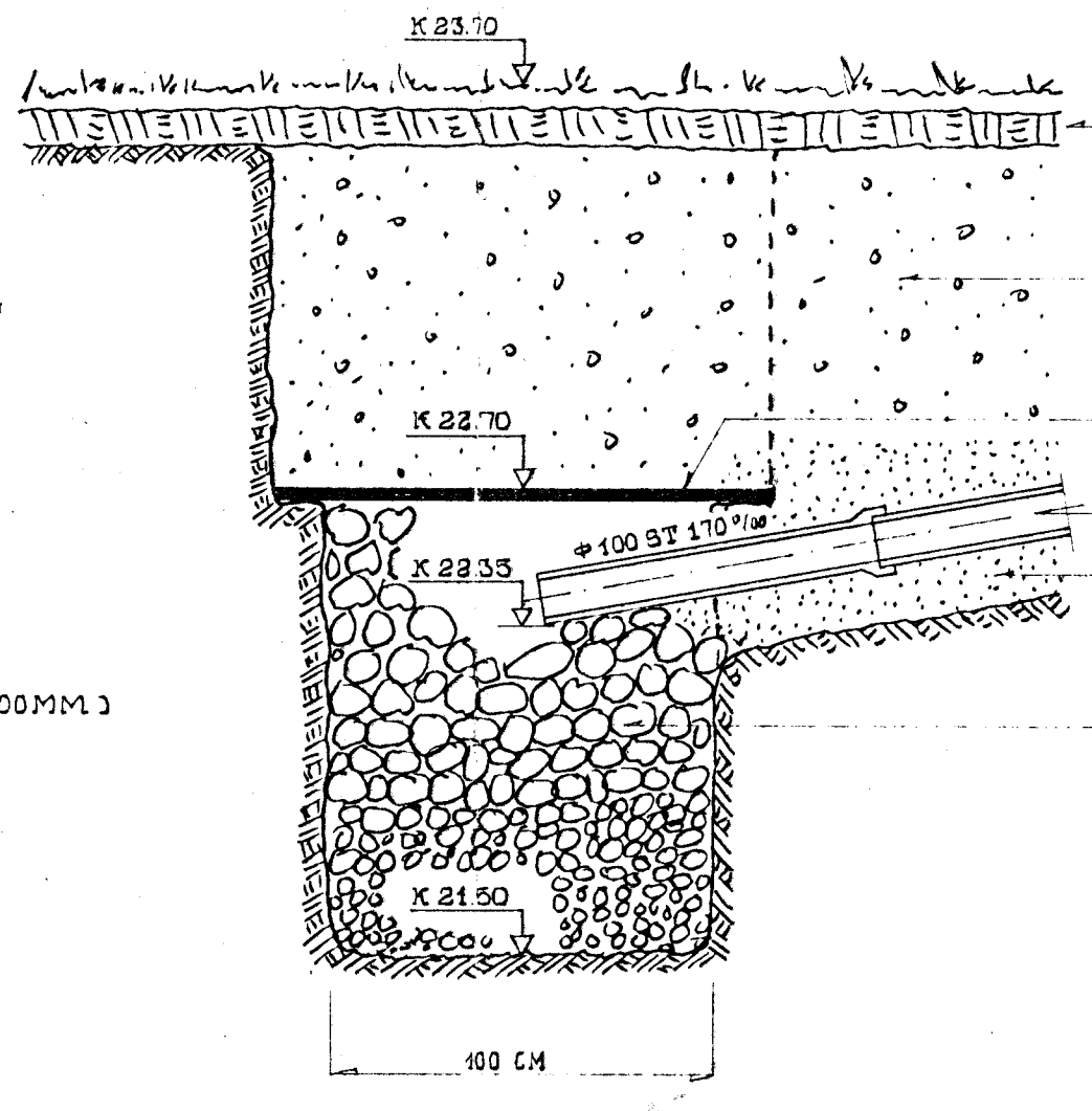
REGNVATNSSVELGUR M=1:20
