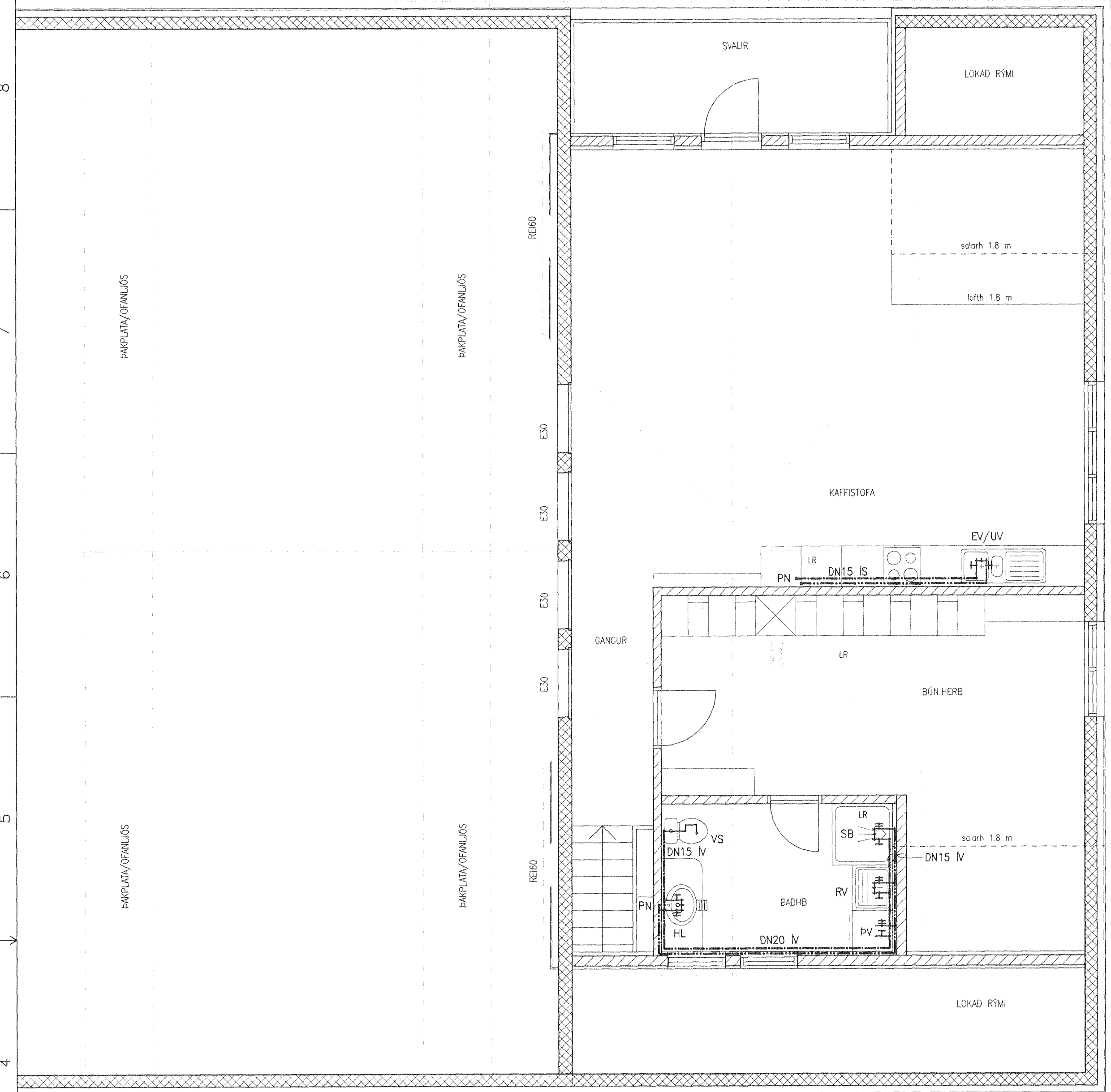
VATNSLÖGN MILLIGÓLF 1:50
