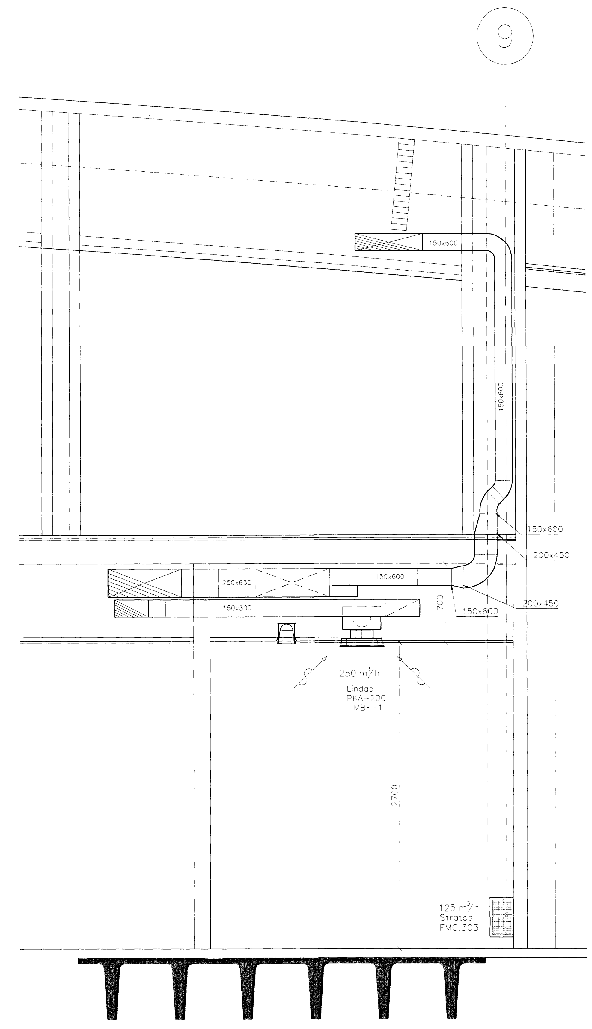
3 2 6 Snið Mkv. 1: 20
