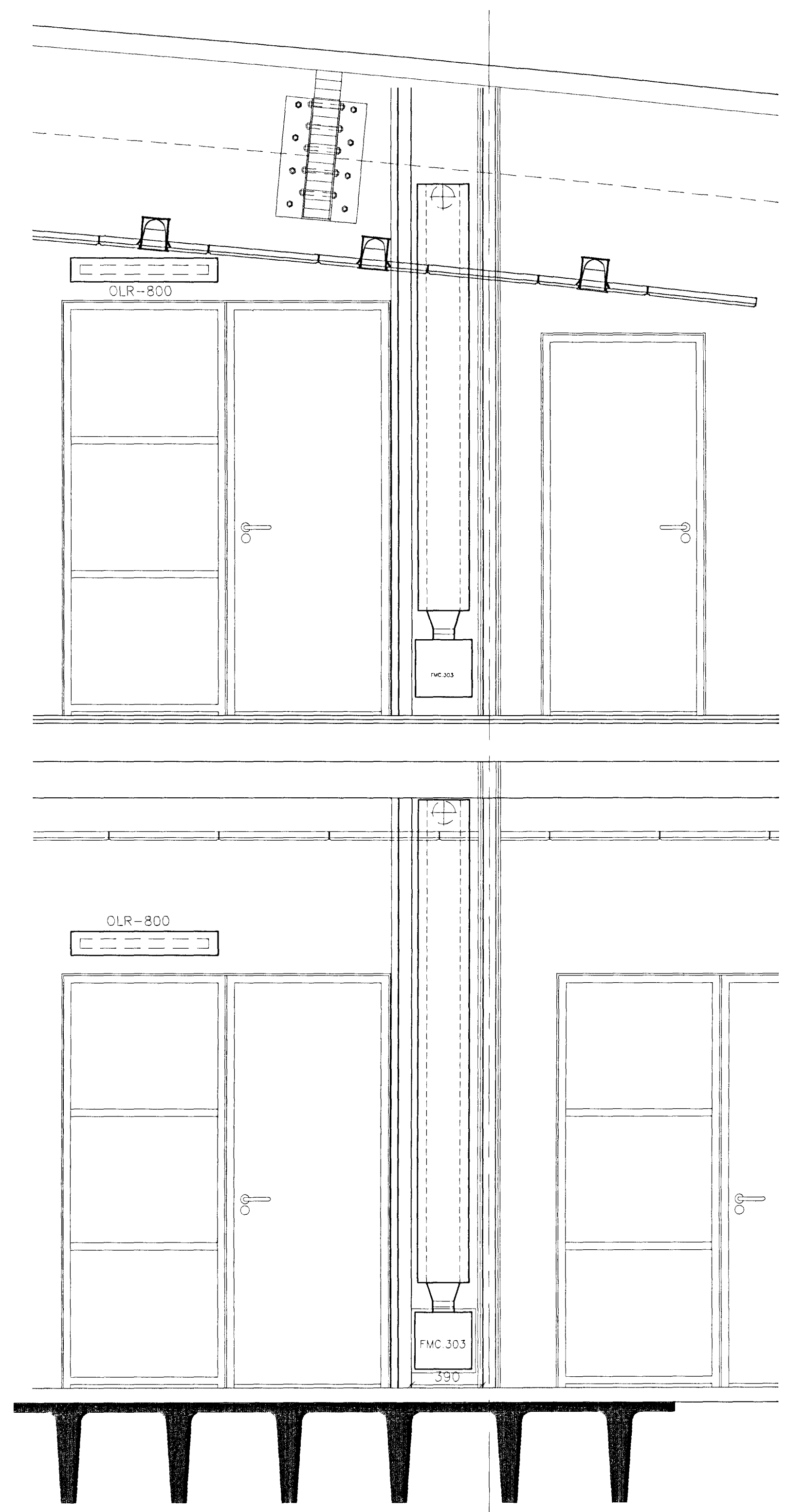
Kennisnið af stökkum og ristum í veggjum Mkv. 1: 20
