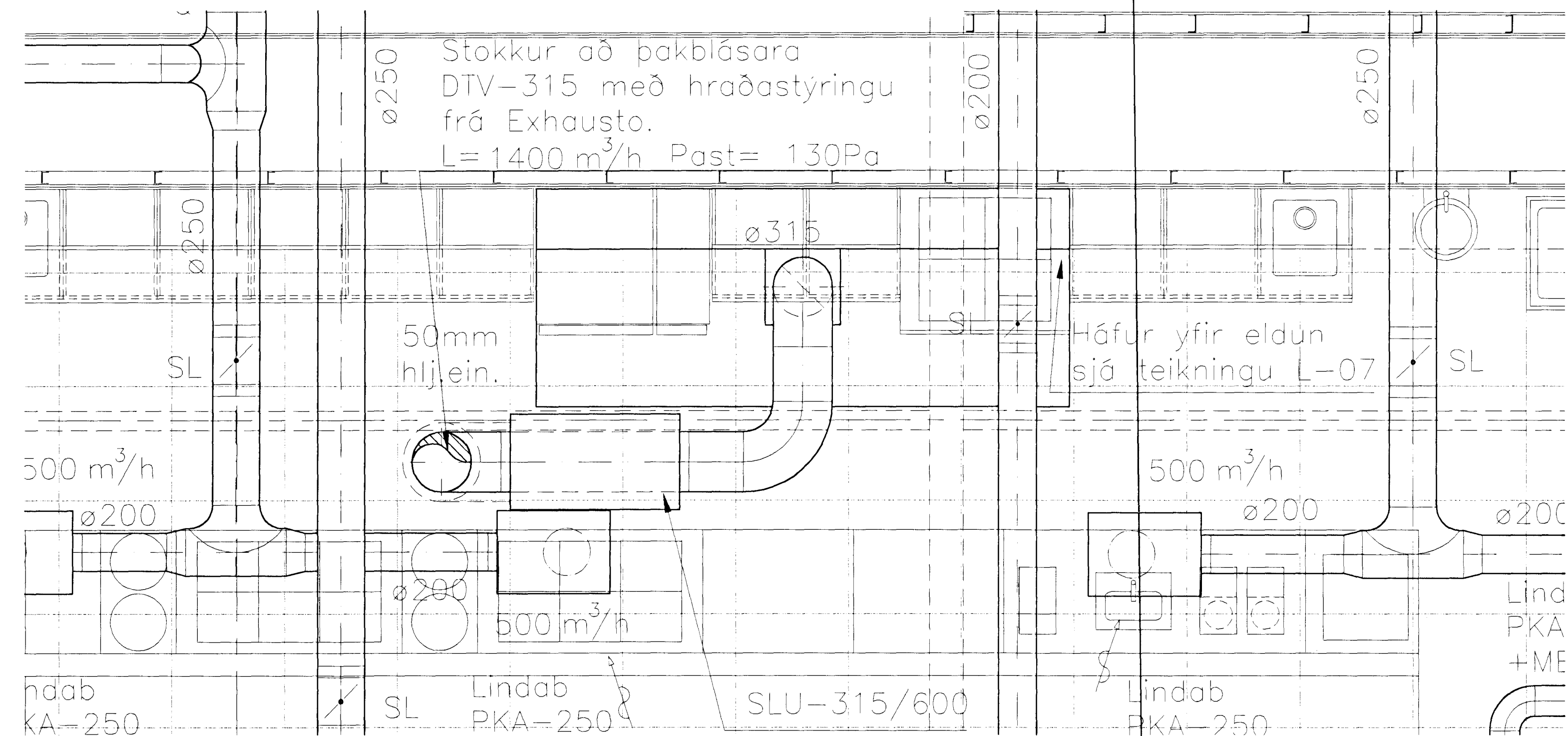
HLUTI ÚR GRUNNMYND 1:20
