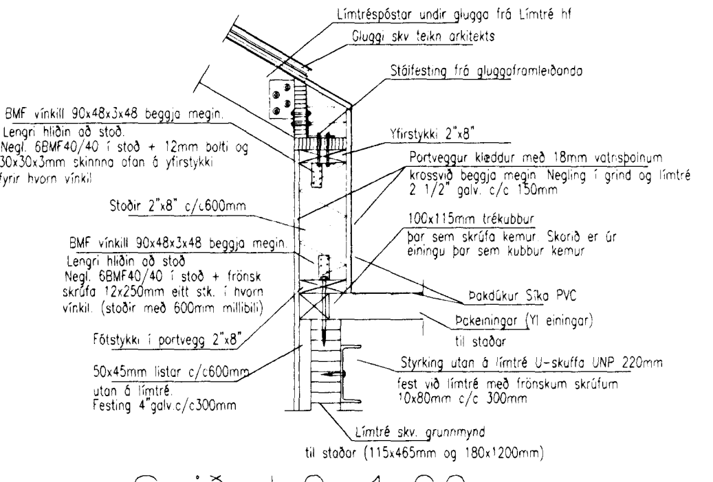
Snið Þ2 1:20
