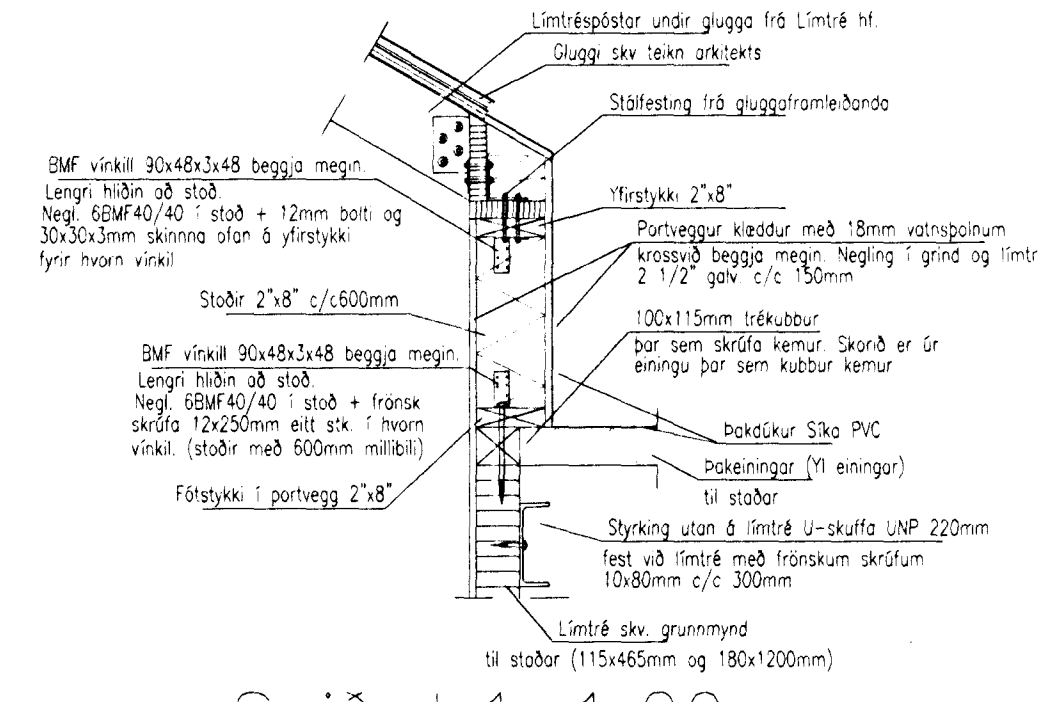
Snið Þ1 1:20
