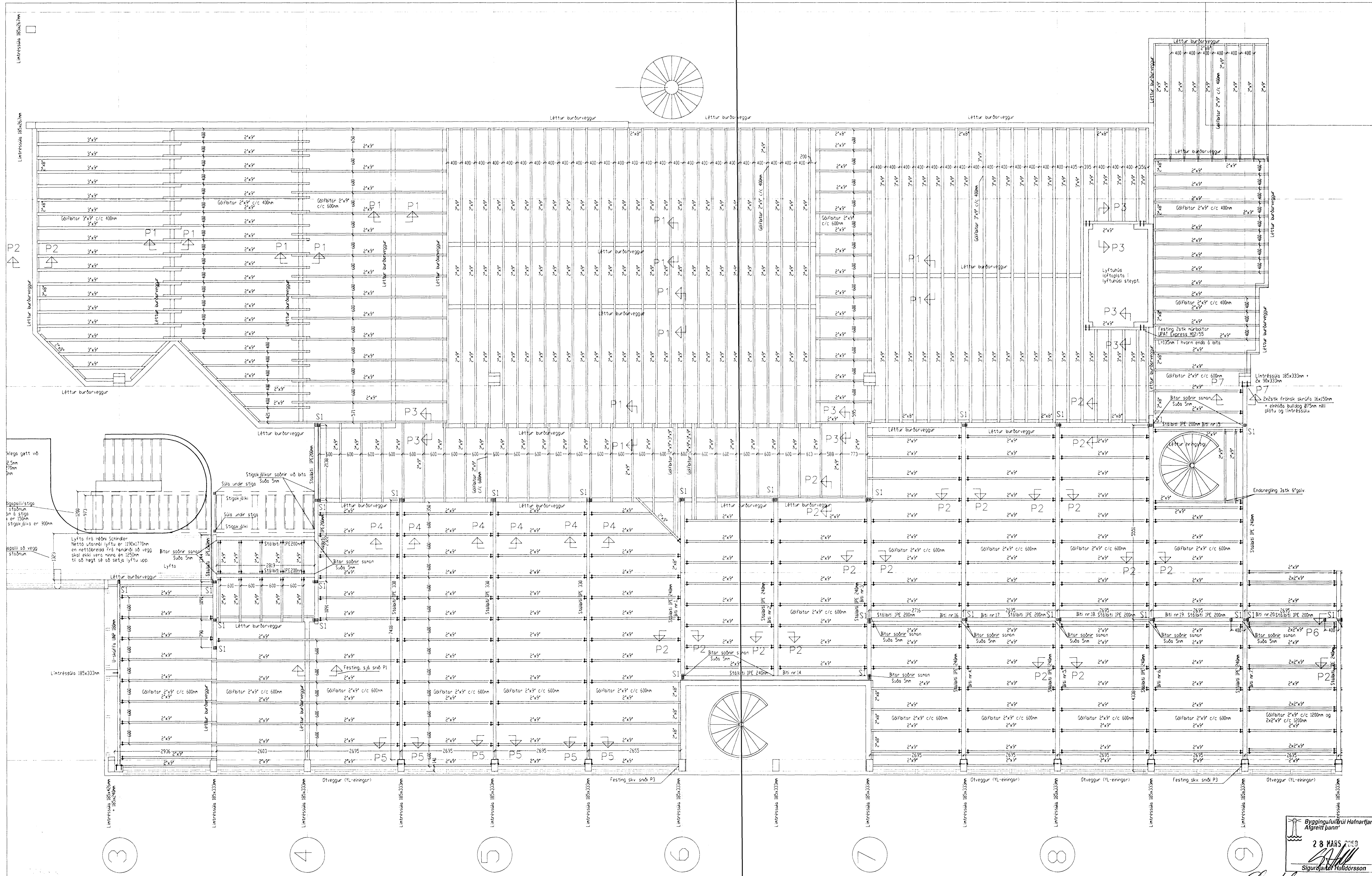
Grunnmynd milliofts 1:50
