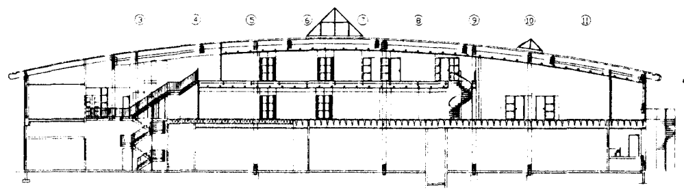
Afstöðumynd/skurður 1:500
