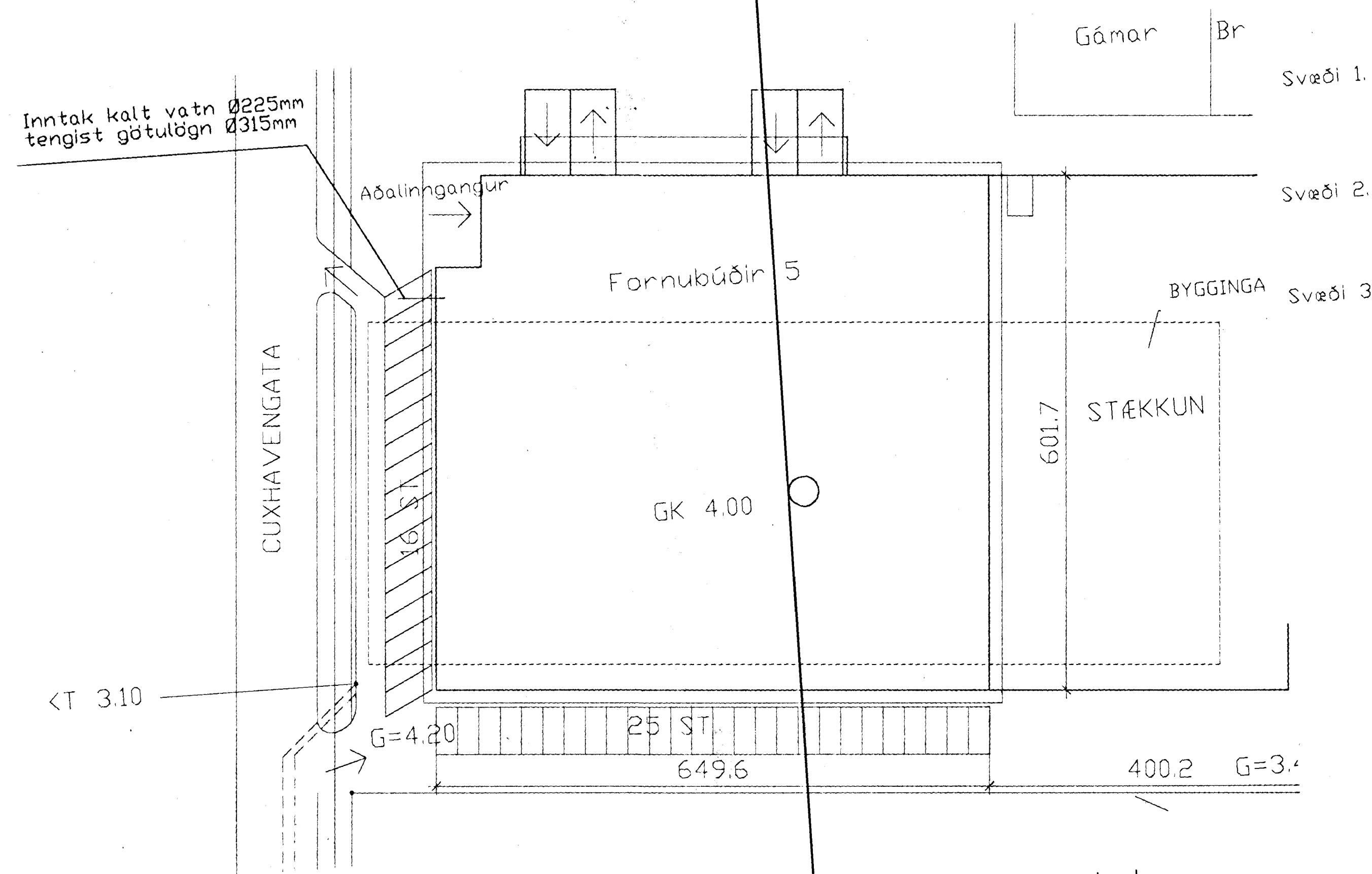
Afstöðumynd af inntaki
