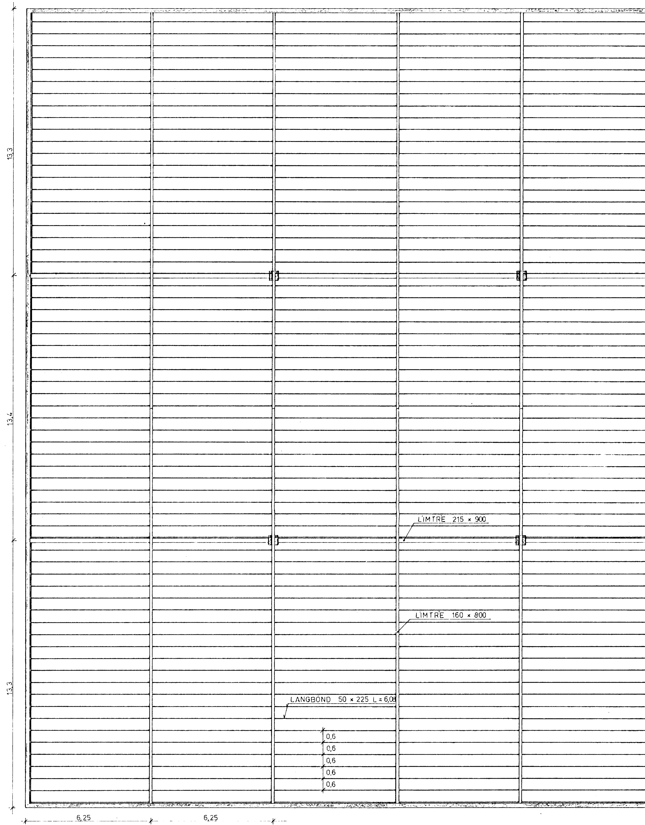
GRUNNMYND 1 : 100
