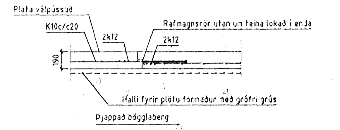
Snið M1 1:25 Snið í þennsluskil
