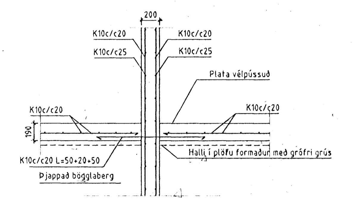
Snið M2 1:25 Snið í steyptan millivegg
