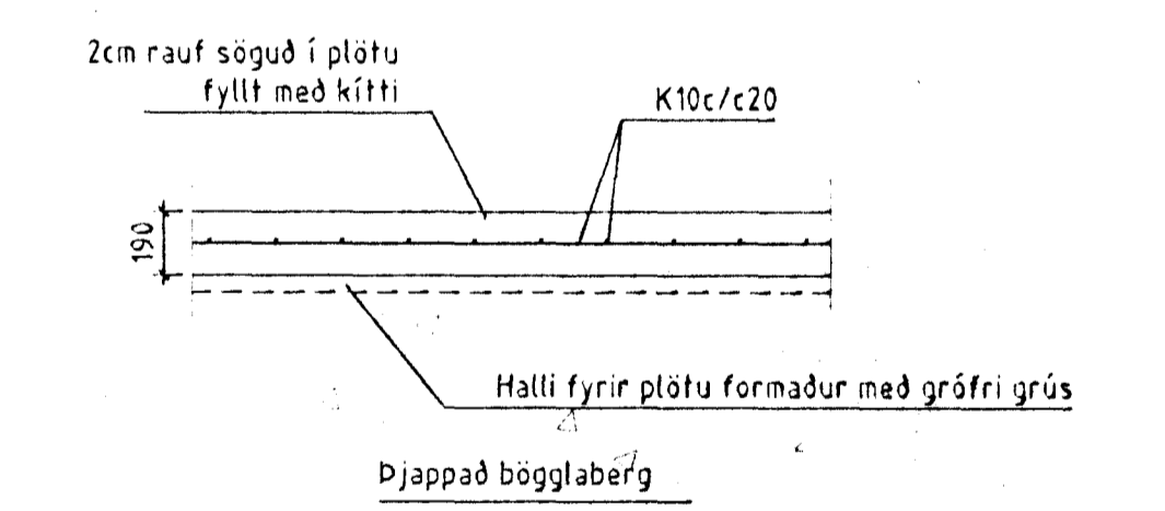
Snið M3 1:25 Snið í steypusögun
