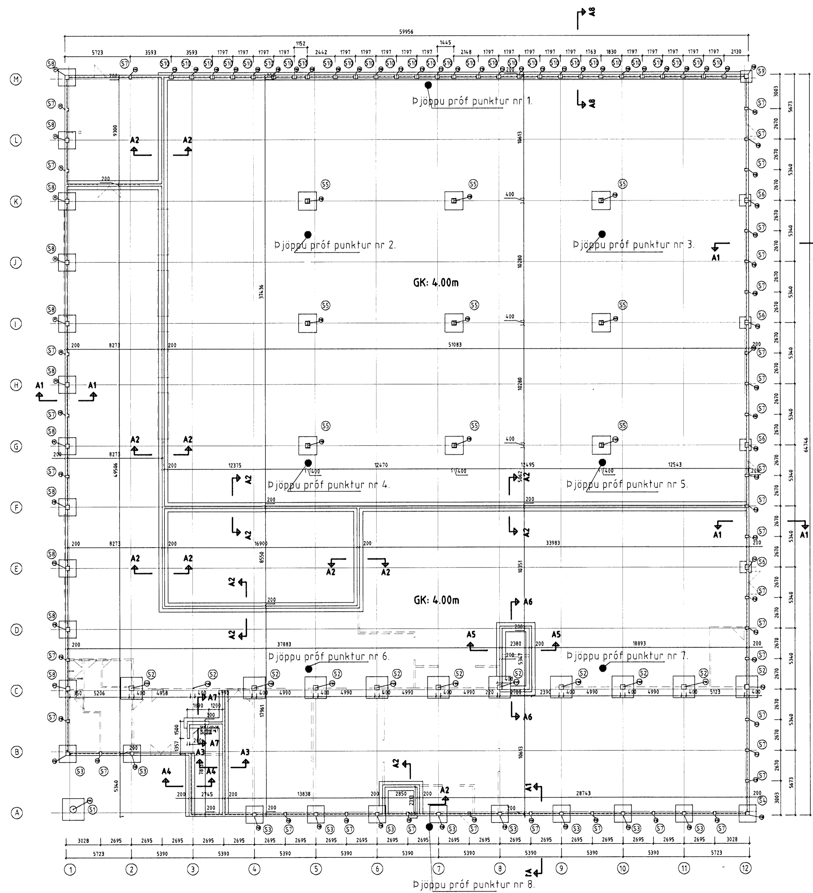
Grunnmynd 1 hæðar 1:200
