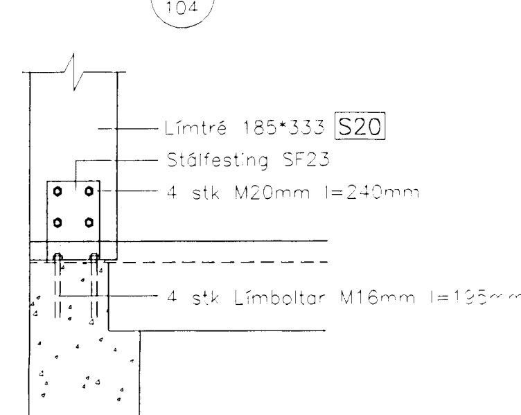
Sérmynd 11 Mkv. 1:20
