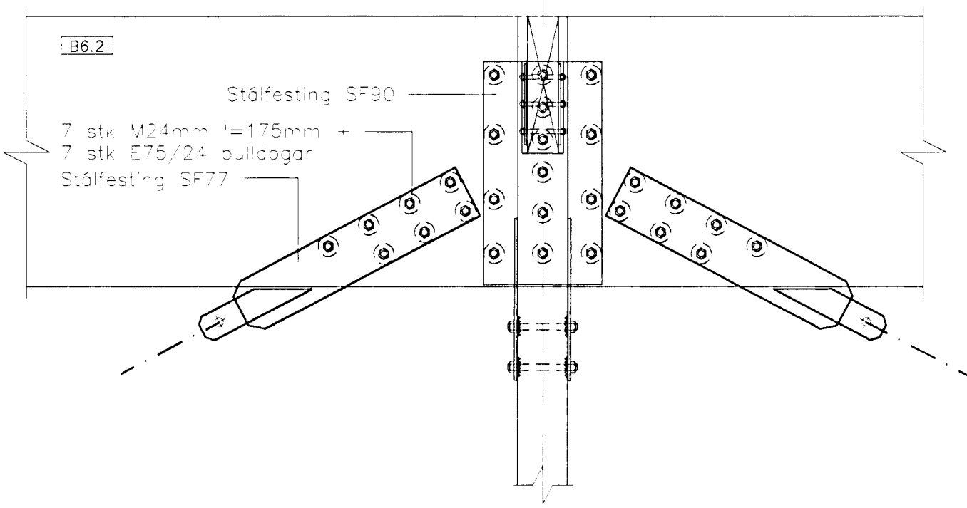
Sérmynd 17 Mkv. 1:20
