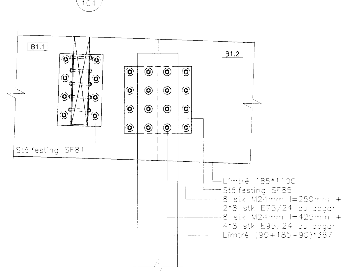
Sérmynd 17 Mkv. 1:20
