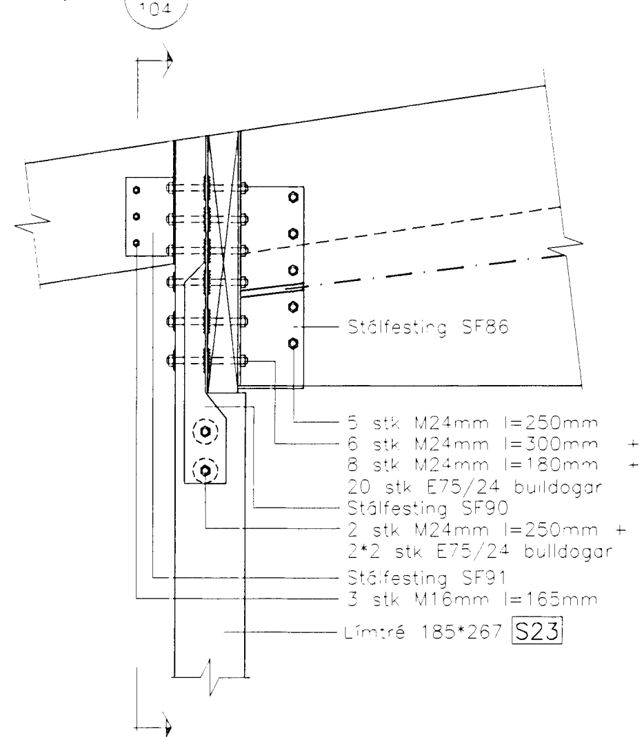
Sérmynd 14 Mkv. 1:20
