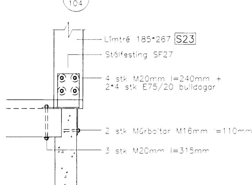
Sérmynd 13 Mkv. 1:20
