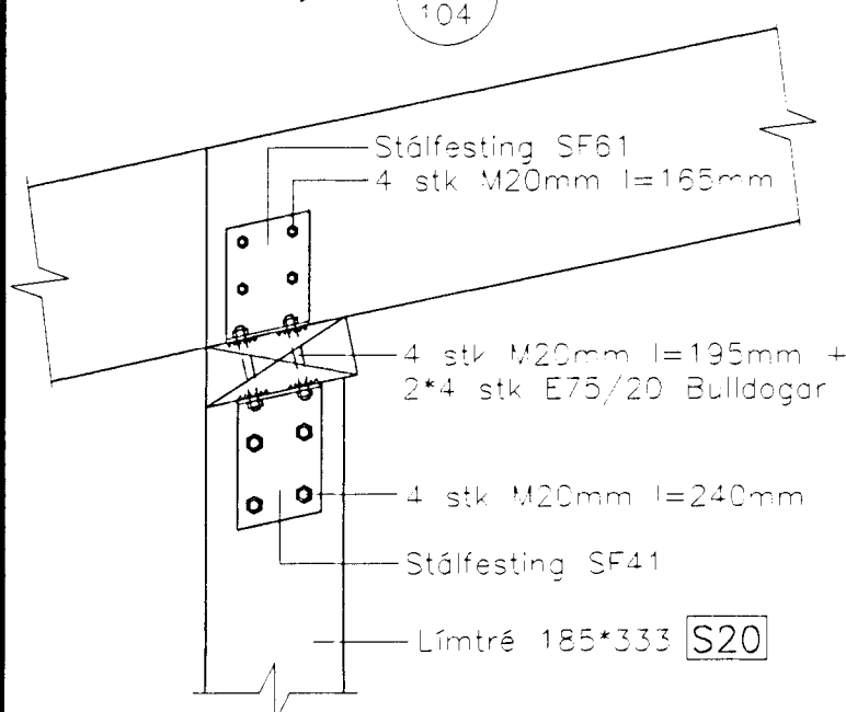
Sérmynd 12 Mkv. 1:20
