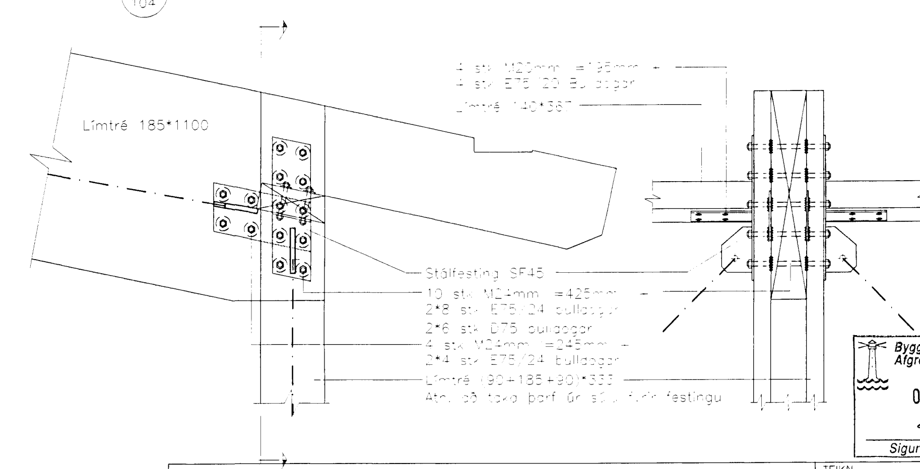
Sérmynd 19 Mkv. 1:20
