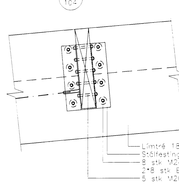
Sérmynd 15 Mkv. 1:20
