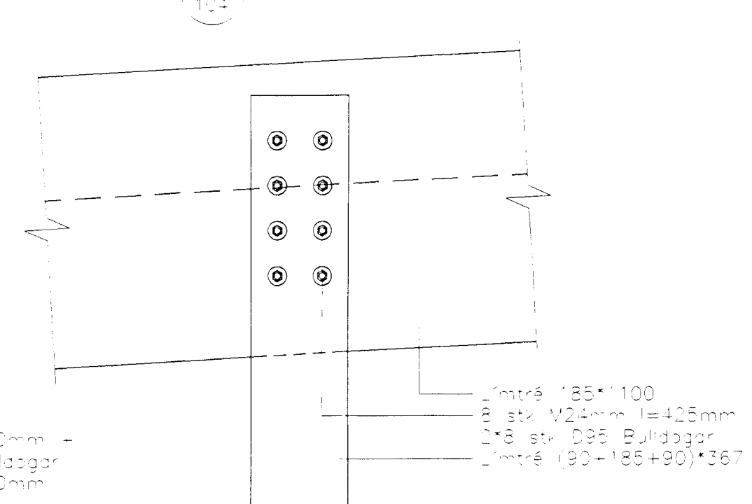
Sérmynd 16 Mkv. 1:20
