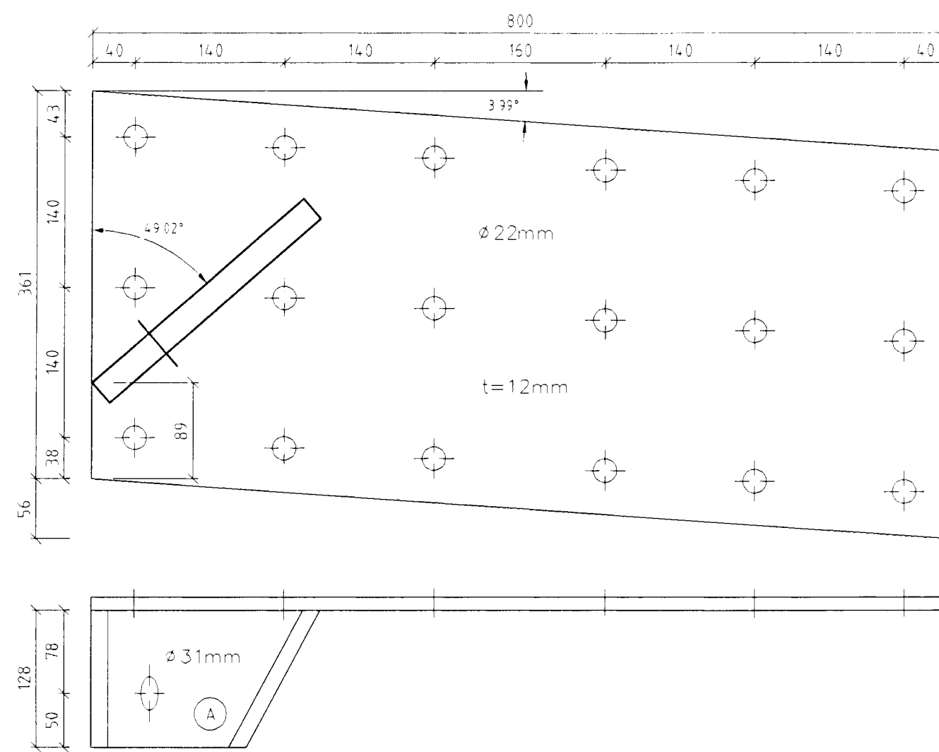
Stálfesting SF55 Mkv. 1:5 Samtals 1 stk
