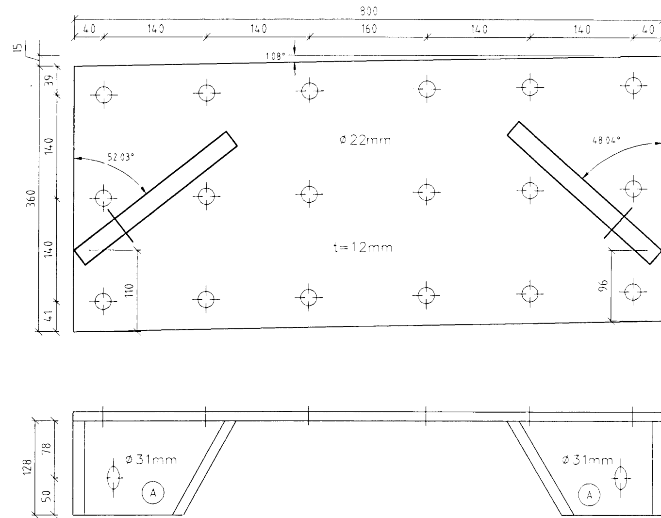
Stálfesting SF54 Mkv. 1:5 Samtals 1 stk
