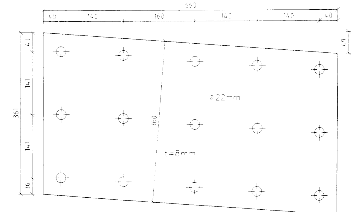
Stálfesting SF59 Mkv. 1:5 Samtals 4 stk
