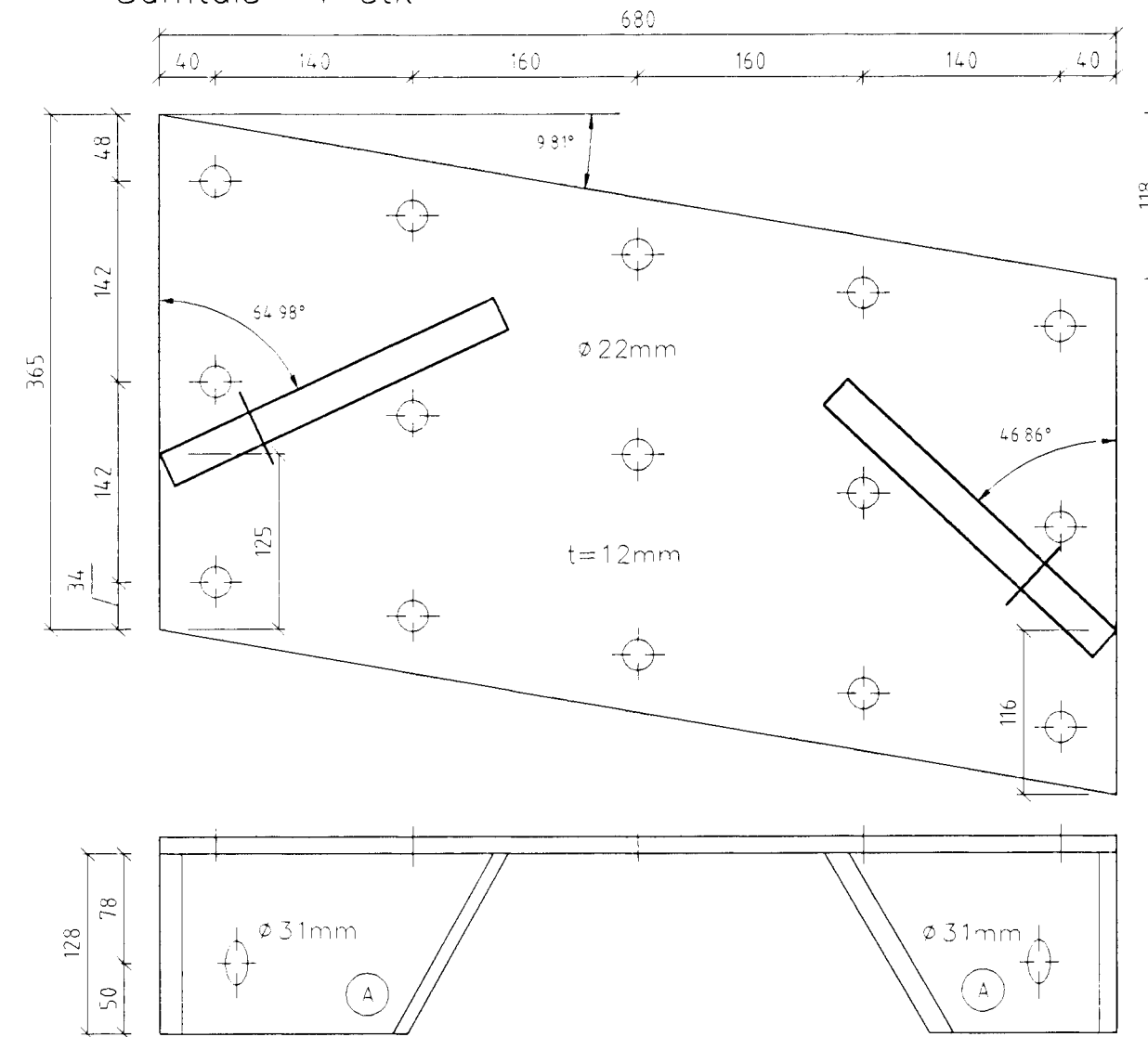
Stálfesting SF57 Mkv. 1:5 Samtals 1 stk
