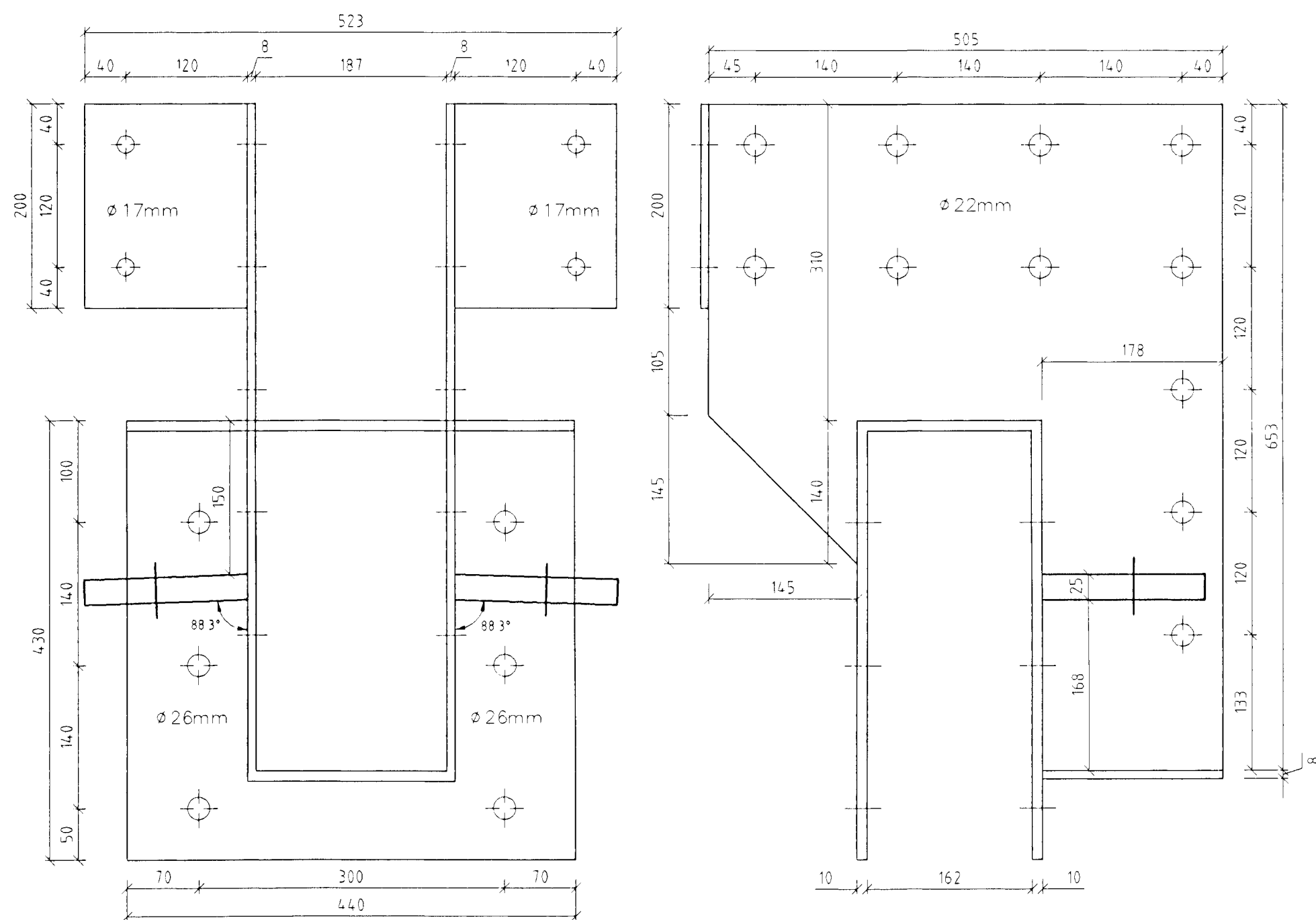
Stálfesting SF56 Mkv. 1:5 Samtals 1 stk
