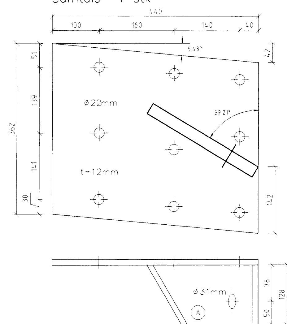
Stálfesting SF56 Mkv. 1:5 Samtals 1 stk
