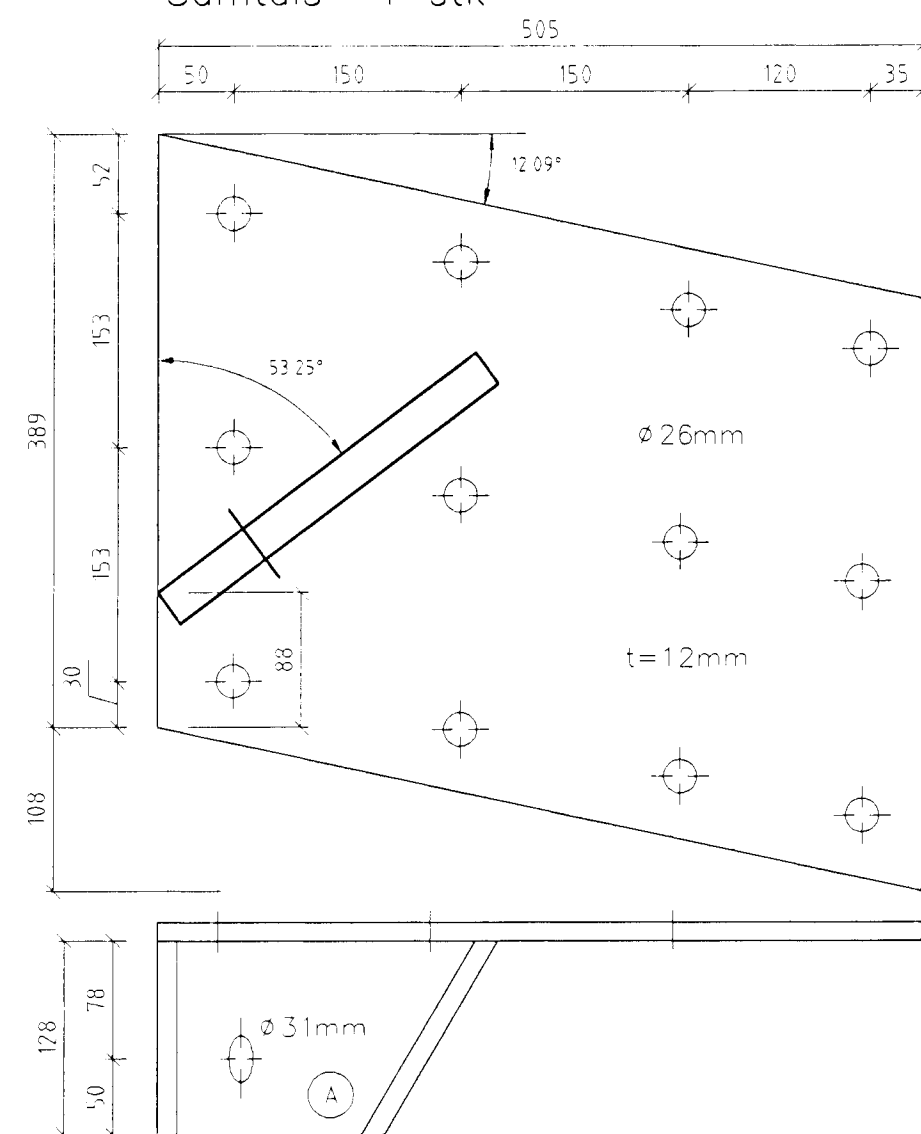
Stálfesting SF58 Mkv. 1:5 Samtals 1 stk
